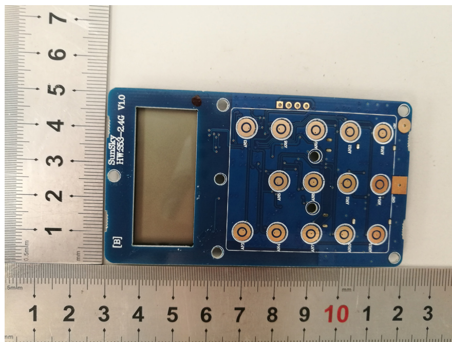
EUT – PCB Bottom View(S53)
