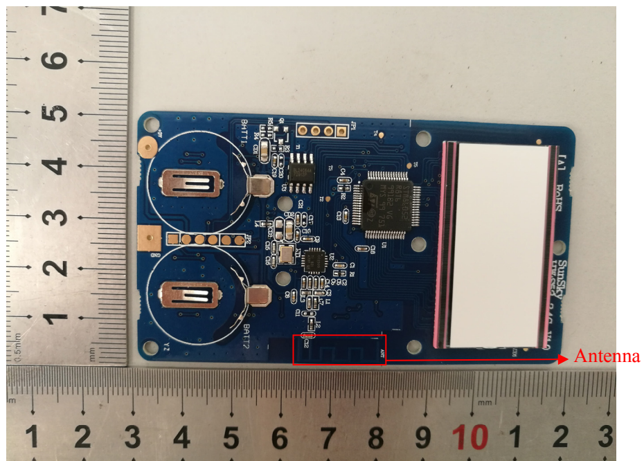
EUT – PCB Bottom View(S53)
