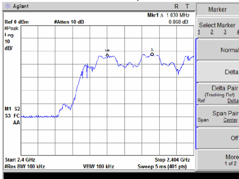
CH00 -3Mbps
