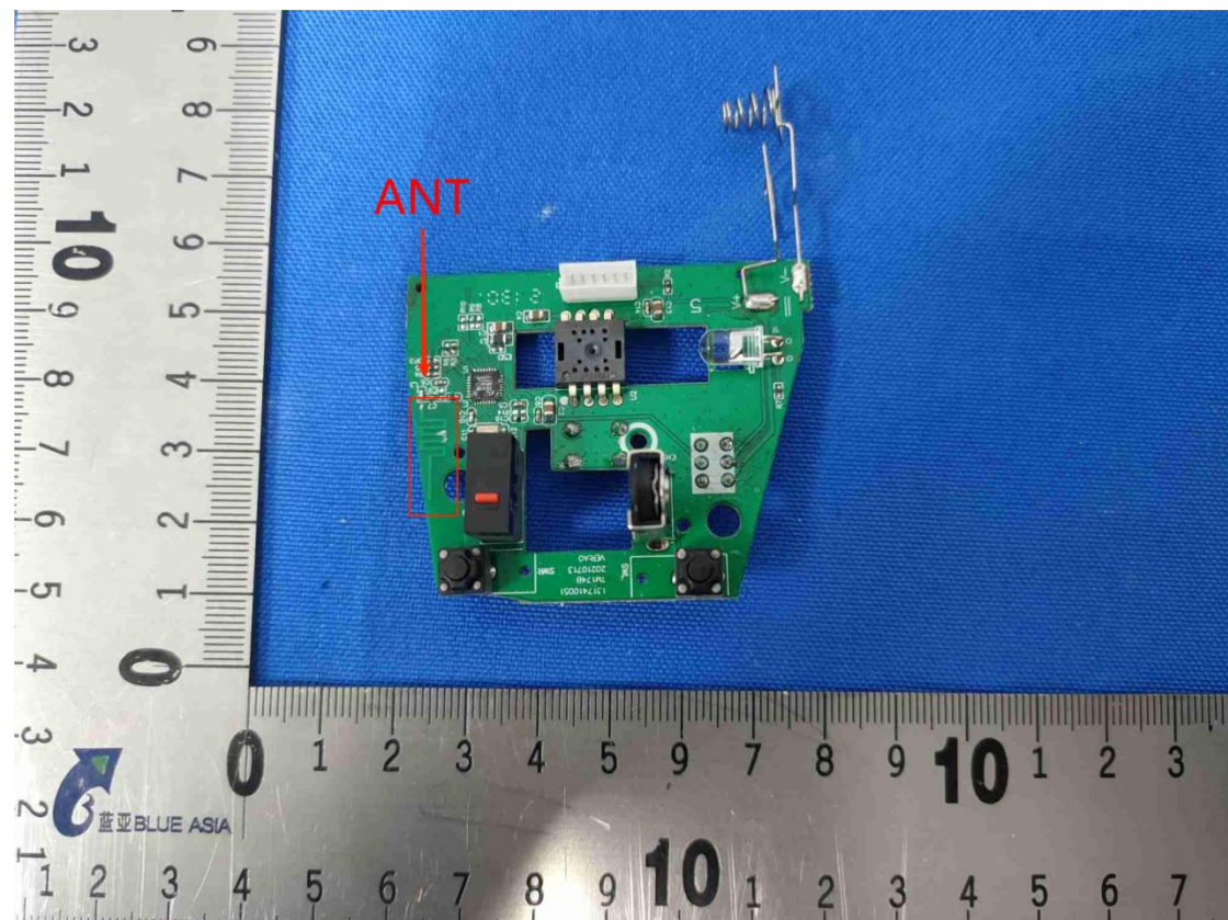
EUT Antenna
