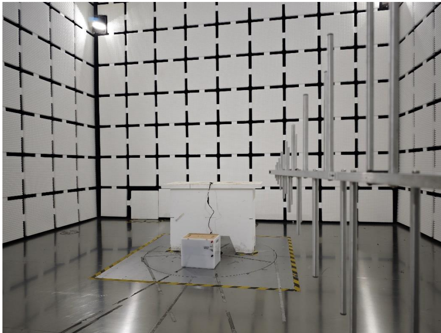
30MHz-1GHz-BT/WIFI
