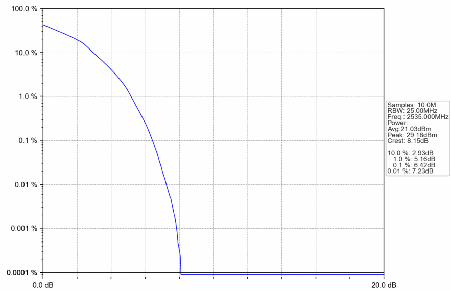
Band7_20MHz_16QAM_MCH_2535MHz_RB_27_0_NTNV
