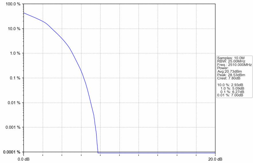
Band7_20MHz_16QAM_LCH_2510MHz_RB_27_0_NTNV
