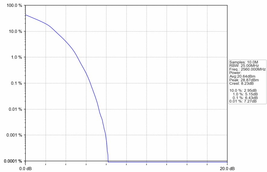
Band7_20MHz_16QAM_HCH_2560MHz_RB_27_73_NTNV
