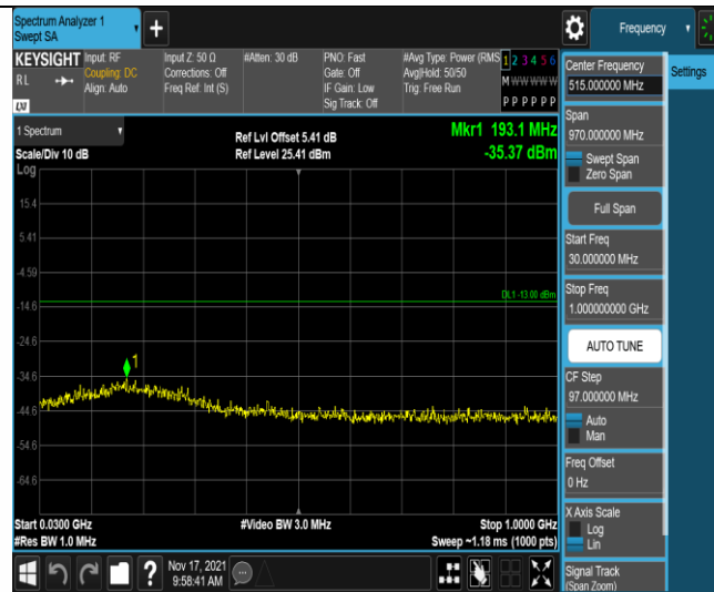
Band4-1.4MHz-QPSK-20393-1RB#0-Range1:30~1000MHz
