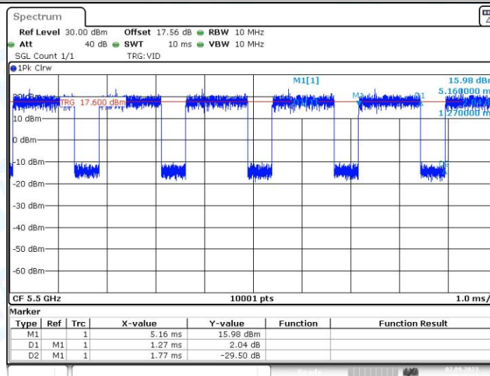
11N20MIMO_Ant1_5500
