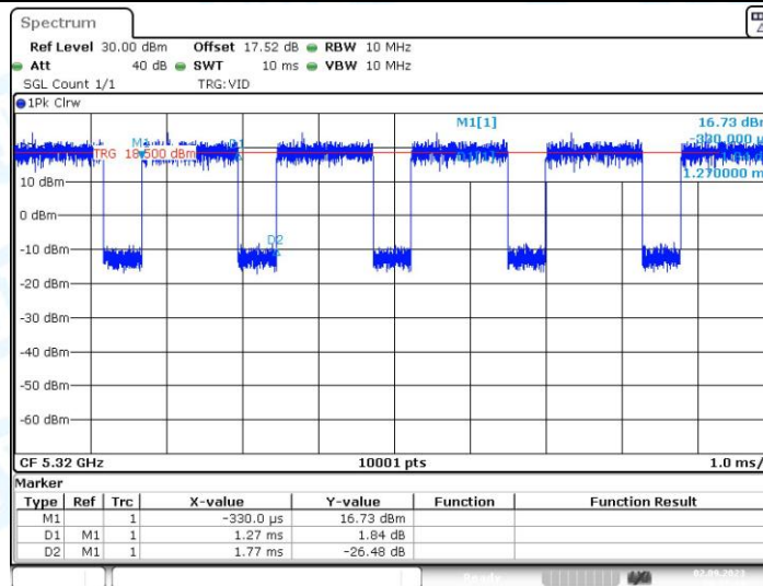
11N20MIMO_Ant2_5320
