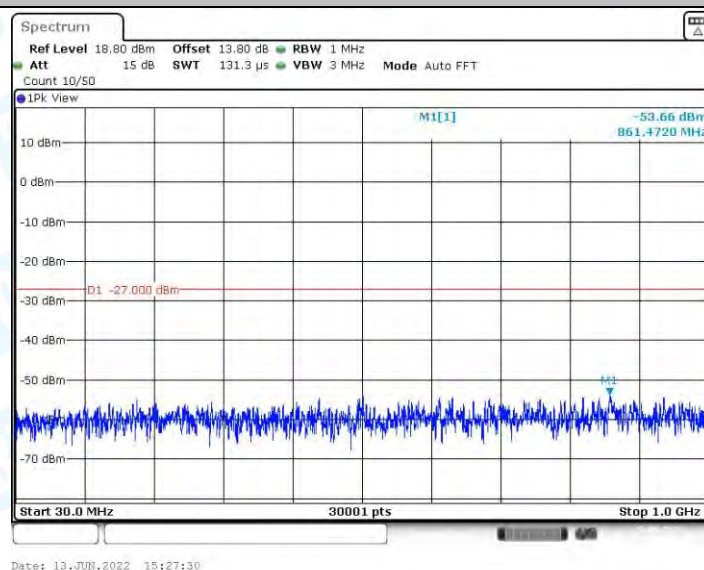
11AC80MIMO_Ant2_5610_30~1000
