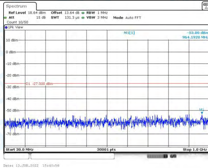
11AX20MIMO_Ant1_5320_30~1000
