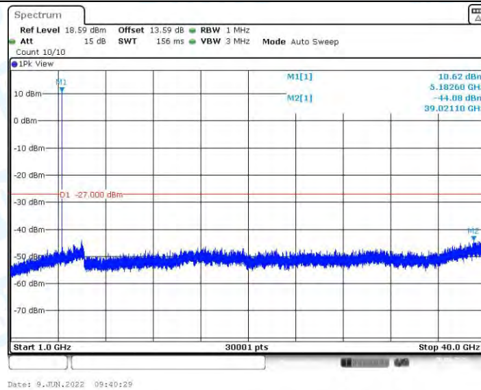
11AX20MIMO_Ant2_5180_1000~40000
