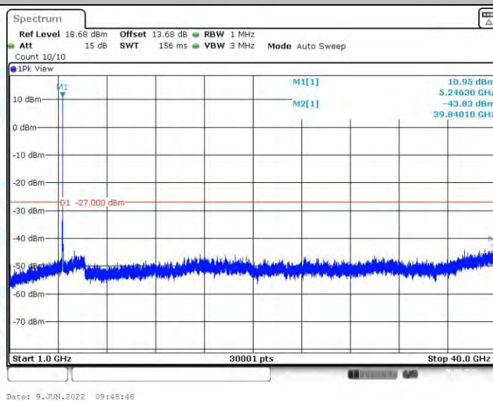
11AX20MIMO_Ant1_5240_1000~40000
