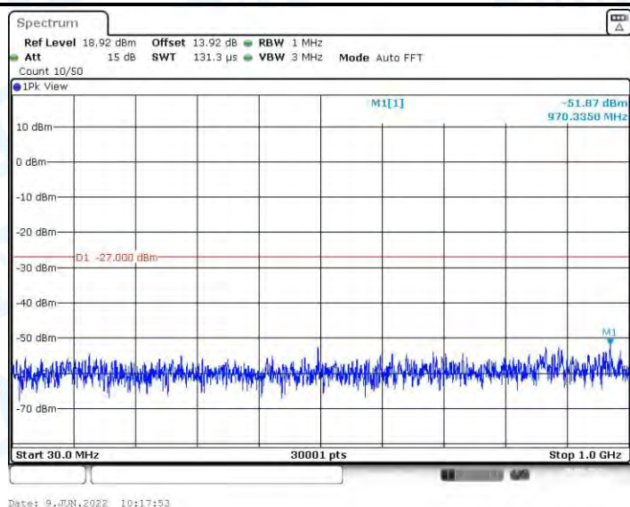
11AX20MIMO_Ant1_5785_30~1000
