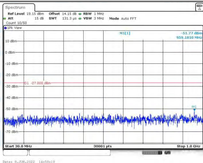
11AC40MIMO_Ant1_5755_30~1000
