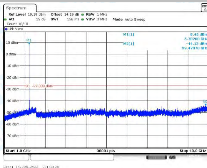
11AX20MIMO_Ant1_5700_1000~40000
