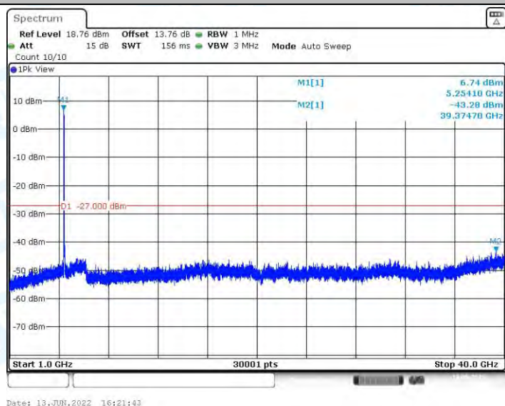
11AX40MIMO_Ant2_5270_1000~40000
