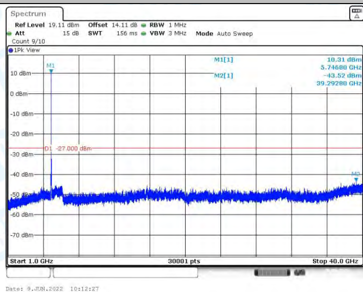
11AX20MIMO_Ant2_5745_1000~40000
