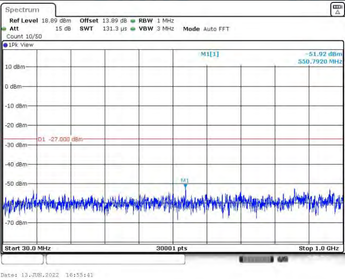
11AX80MIMO_Ant2_5290_30~1000
