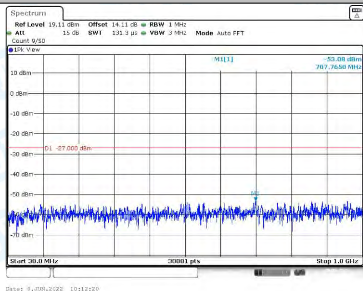
11AX20MIMO_Ant2_5745_30~1000
