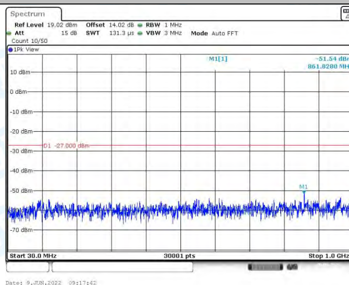
11AC80MIMO_Ant1_5775_30~1000
