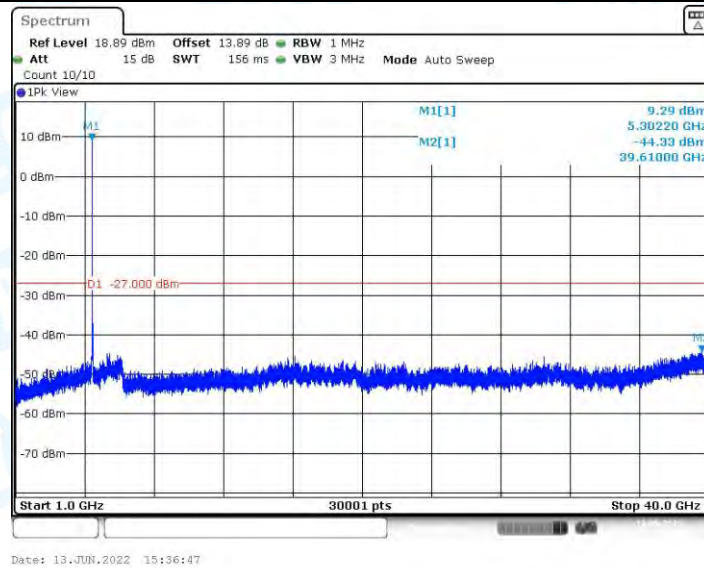
11AX20MIMO_Ant2_5300_1000~40000
