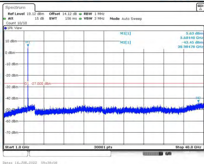
11AX40MIMO_Ant1_5670_1000~40000
