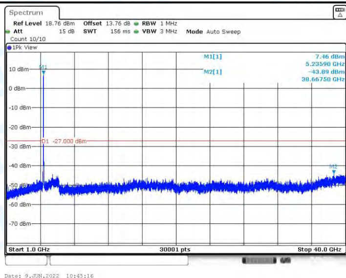
11AX40MIMO_Ant2_5230_1000~40000
