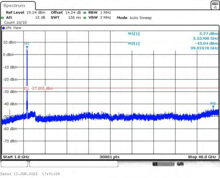
11AX80MIMO_Ant1_5530_1000~40000
