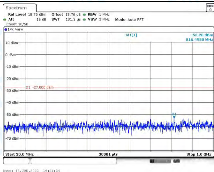
11AX40MIMO_Ant2_5270_30~1000
