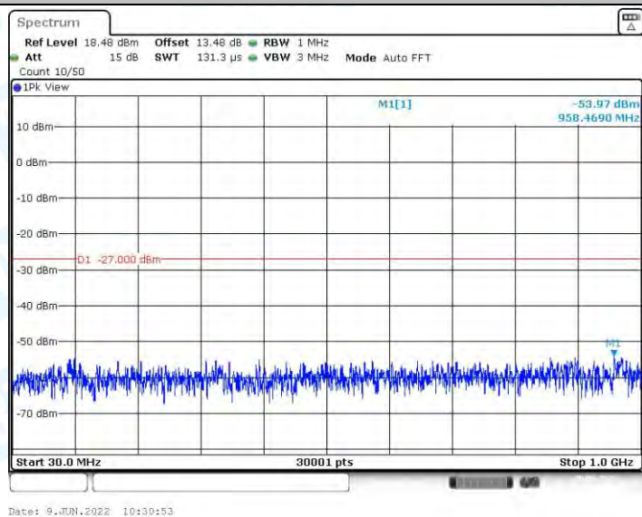
11AX40MIMO_Ant1_5190_30~1000
