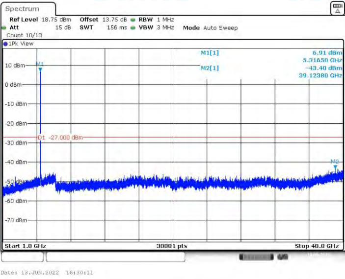
11AX40MIMO_Ant2_5310_1000~40000
