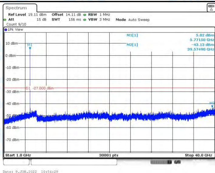
11AX40MIMO_Ant2_5755_1000~40000
