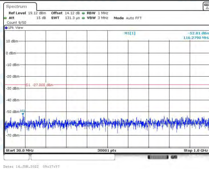
11AX40MIMO_Ant1_5670_30~1000
