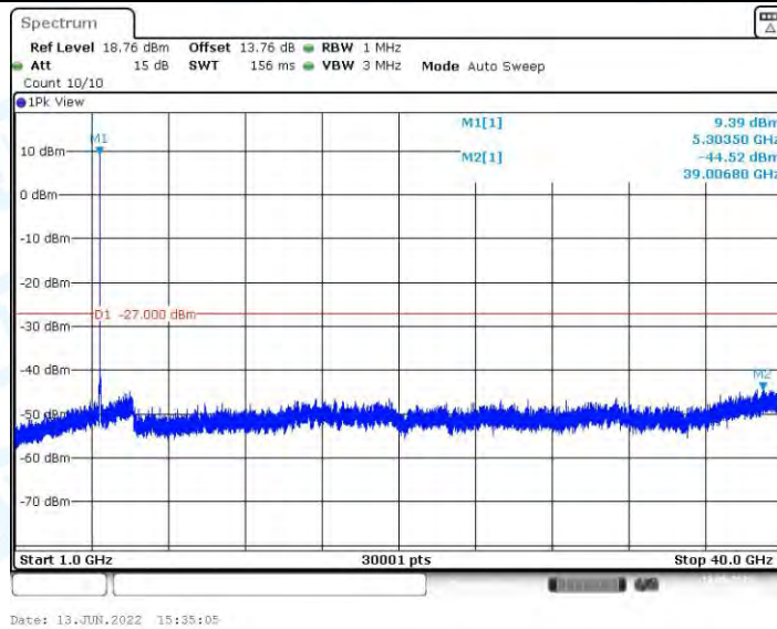
11AX20MIMO_Ant1_5300_1000~40000
