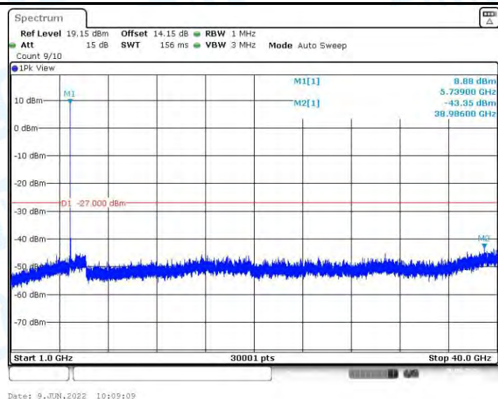
11AX20MIMO_Ant1_5745_1000~40000
