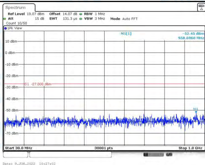
11AX20MIMO_Ant2_5825_30~1000
