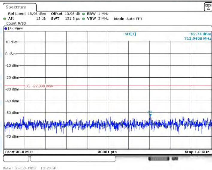
11AX20MIMO_Ant1_5825_30~1000
