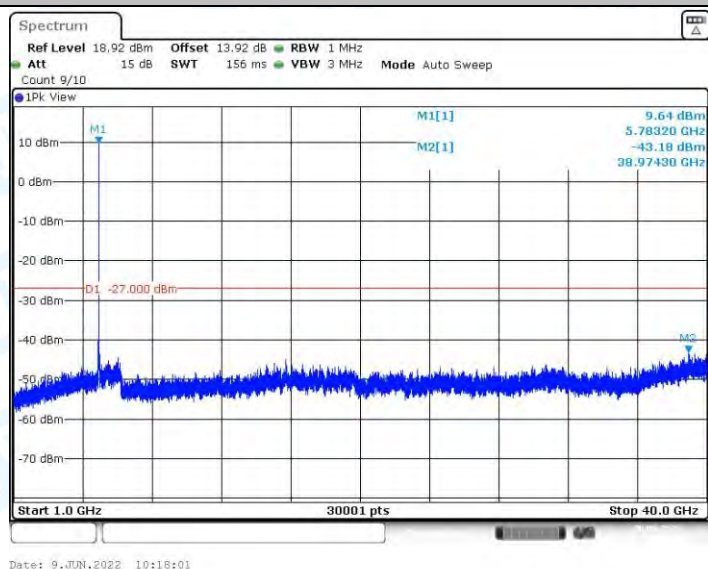
11AX20MIMO_Ant1_5785_1000~40000
