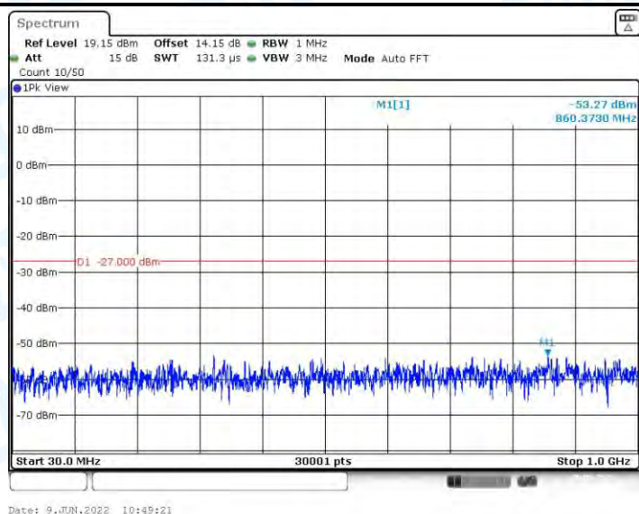
11AX40MIMO_Ant1_5755_30~1000
