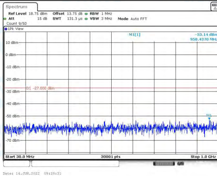
11AX20MIMO_Ant1_5260_30~1000
