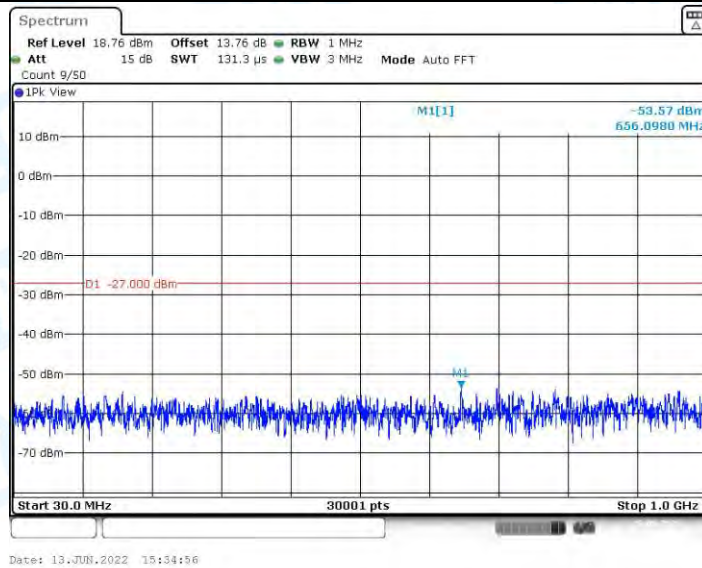
11AX20MIMO_Ant1_5300_30~1000
