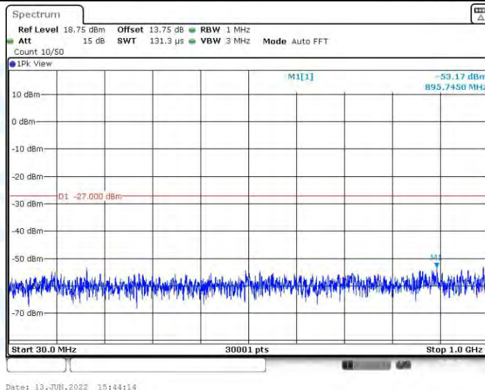
11AX20MIMO_Ant2_5320_30~1000
