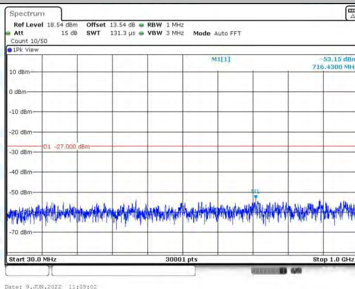
11AX80MIMO_Ant1_5210_30~1000
