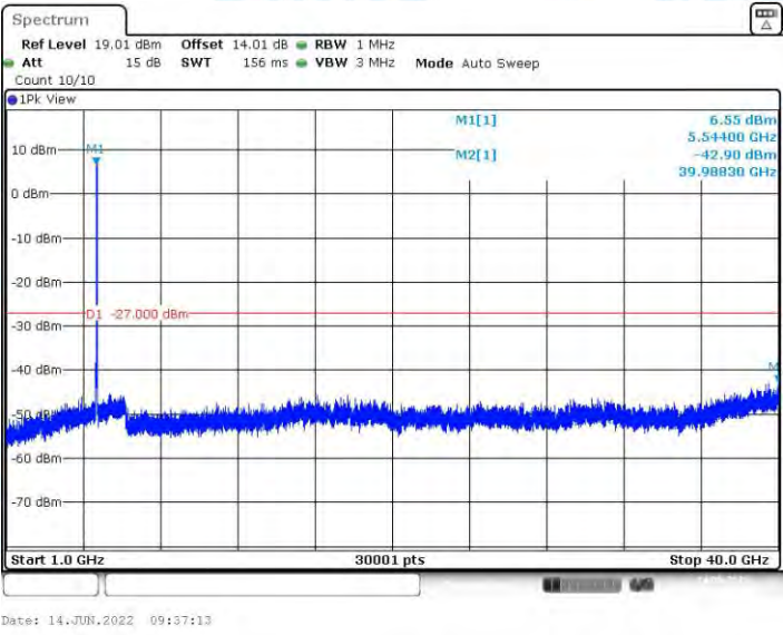
11AX40MIMO_Ant1_5550_1000~40000
