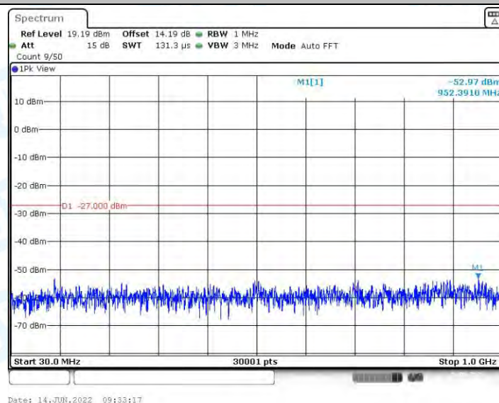
11AX20MIMO_Ant1_5700_30~1000
