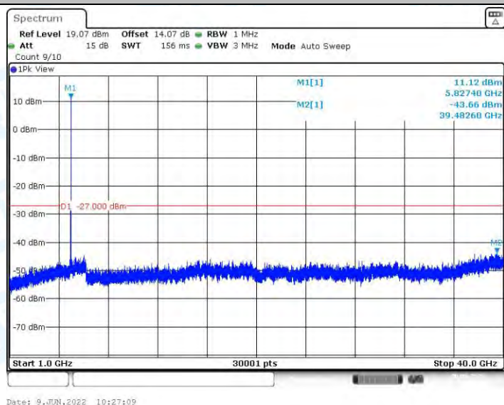
11AX20MIMO_Ant2_5825_1000~40000
