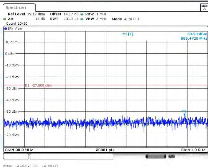
11AX20MIMO_Ant2_5500_30~1000
