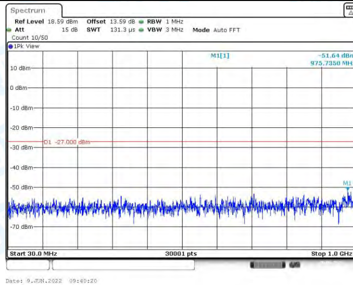
11AX20MIMO_Ant2_5180_30~1000
