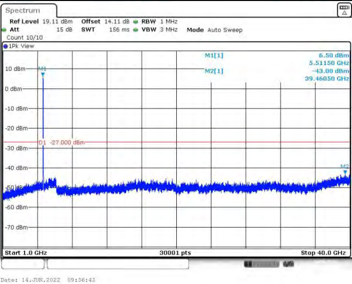
11AX40MIMO_Ant2_5510_1000~40000
