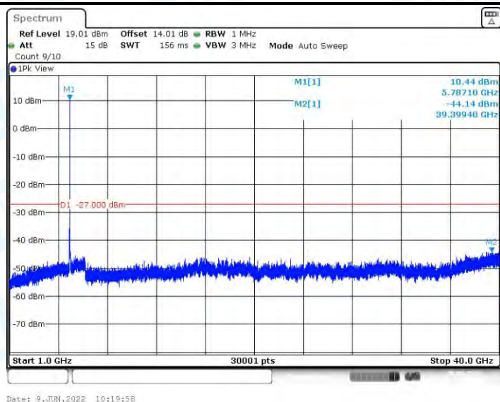
11AX20MIMO_Ant2_5785_1000~40000
