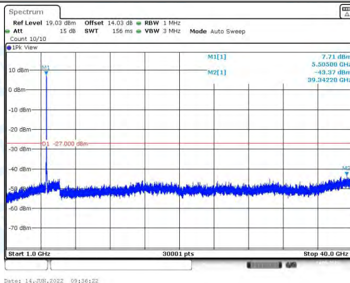
11AX40MIMO_Ant1_5510_1000~40000
