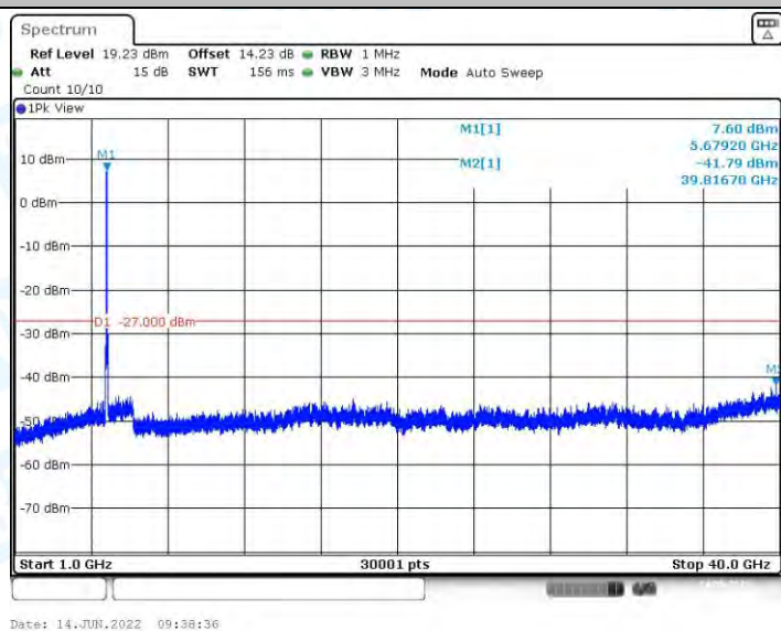
11AX40MIMO_Ant2_5670_1000~40000
