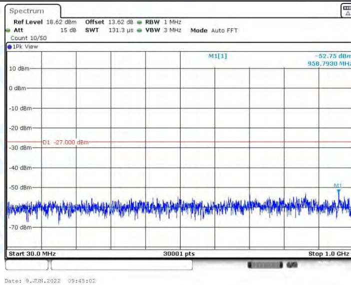
11AX20MIMO_Ant2_5220_30~1000
