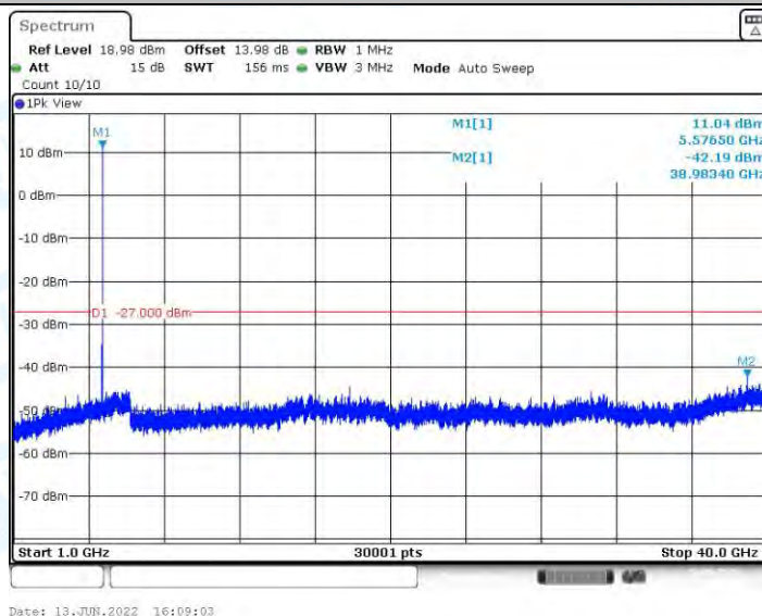
11AX20MIMO_Ant1_5580_1000~40000
