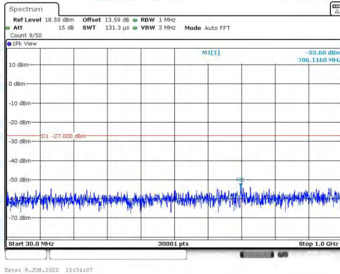
11AX40MIMO_Ant2_5190_30~1000
