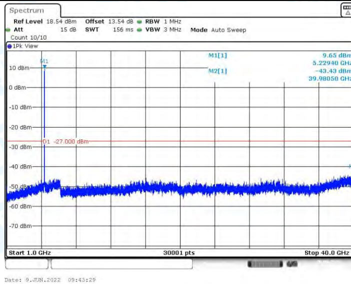
11AX20MIMO_Ant1_5220_1000~40000
