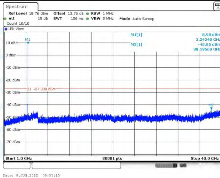
11AX20MIMO_Ant2_5240_1000~40000
