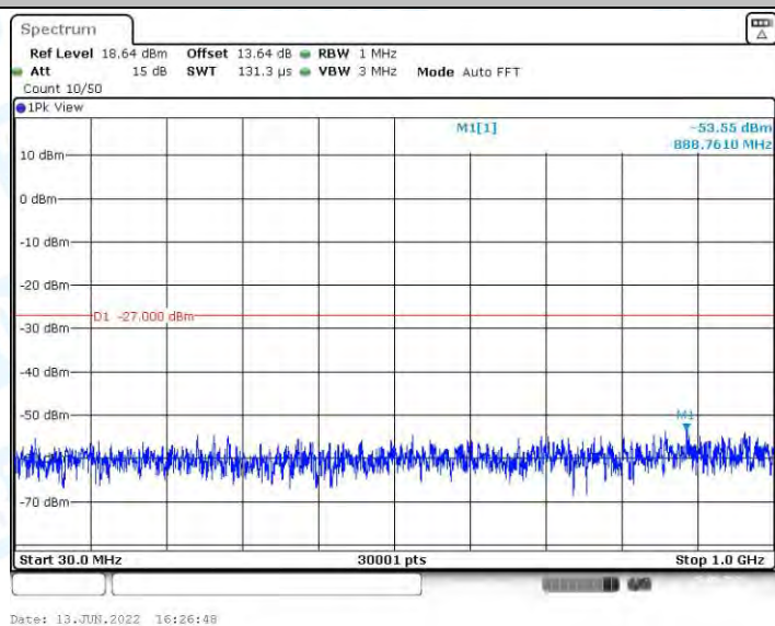
11AX40MIMO_Ant1_5310_30~1000
