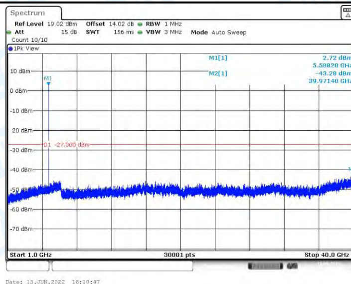
11AX20MIMO_Ant2_5580_1000~40000
