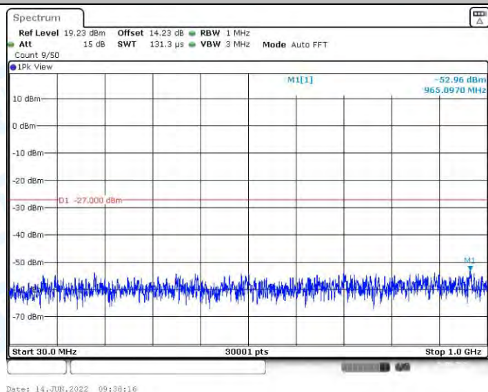
11AX40MIMO_Ant2_5670_30~1000
