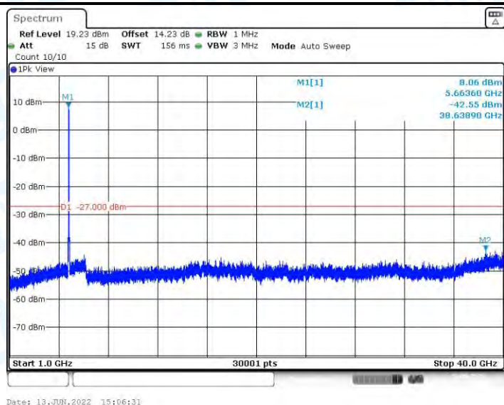
11AC40MIMO_Ant2_5670_1000~40000
