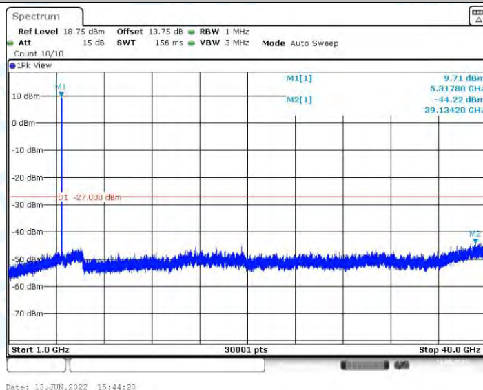
11AX20MIMO_Ant2_5320_1000~40000
