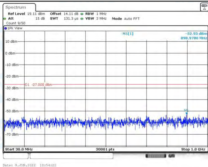
11AX40MIMO_Ant2_5755_30~1000
