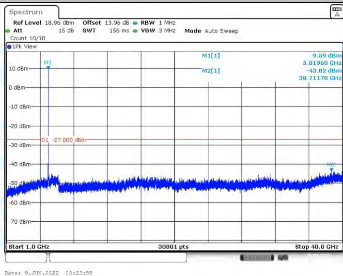
11AX20MIMO_Ant1_5825_1000~40000
