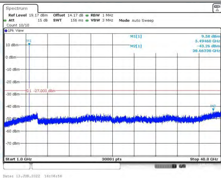
11AX20MIMO_Ant2_5500_1000~40000
