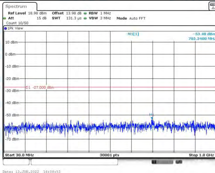
11AX20MIMO_Ant1_5580_30~1000
