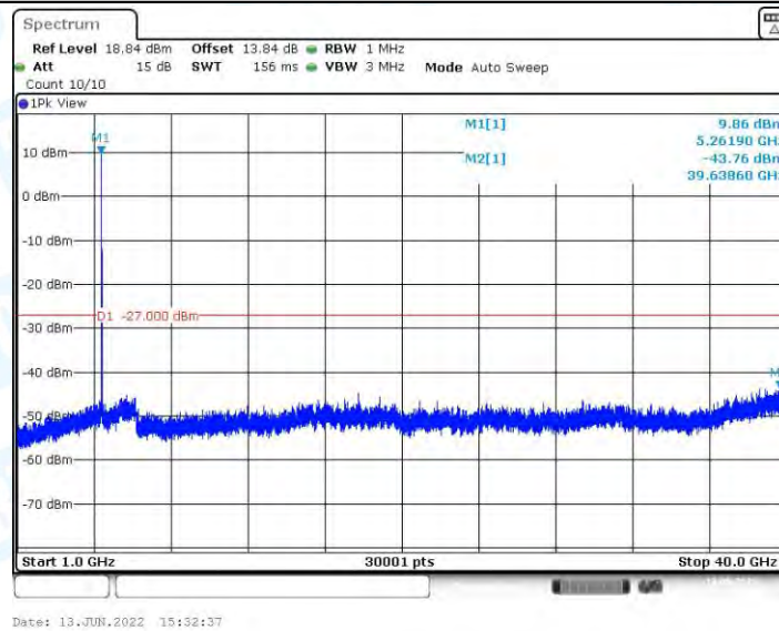
11AX20MIMO_Ant2_5260_1000~40000
