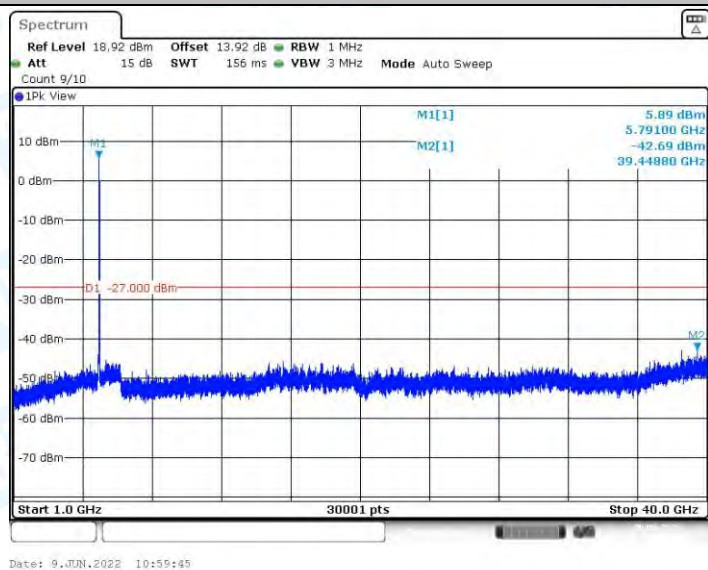
11AX40MIMO_Ant1_5795_1000~40000
