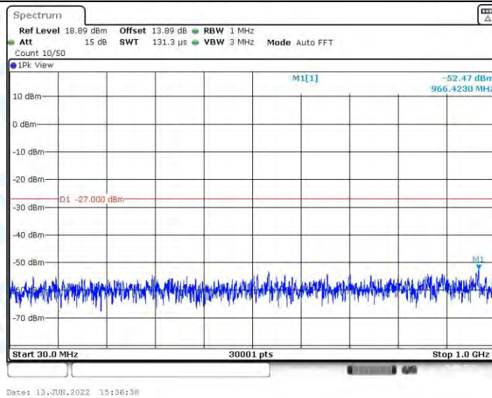
11AX20MIMO_Ant2_5300_30~1000
