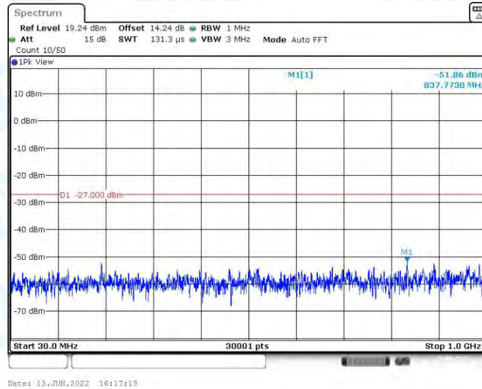
11AX20MIMO_Ant2_5700_30~1000
