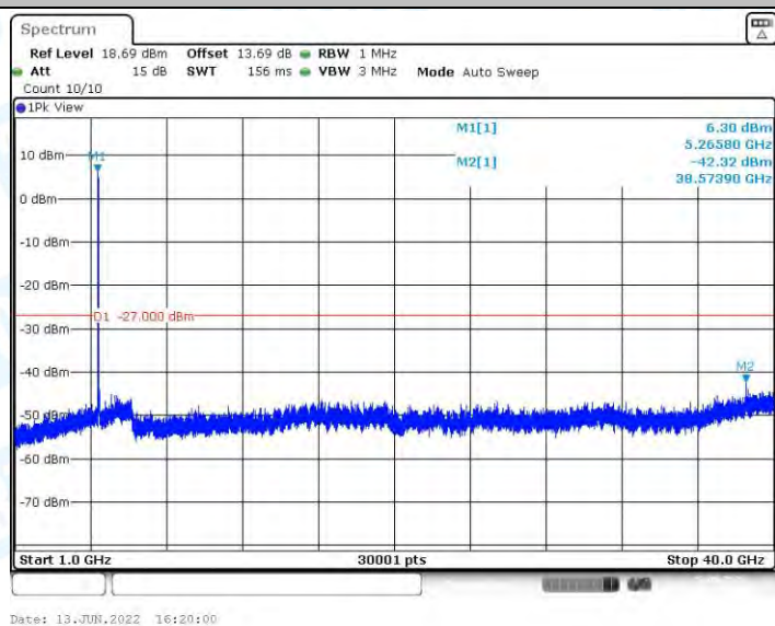
11AX40MIMO_Ant1_5270_1000~40000
