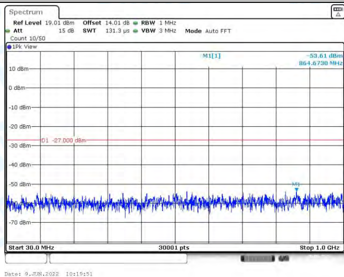
11AX20MIMO_Ant2_5785_30~1000
