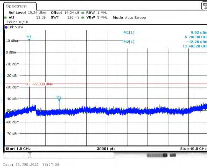
11AX20MIMO_Ant2_5700_1000~40000
