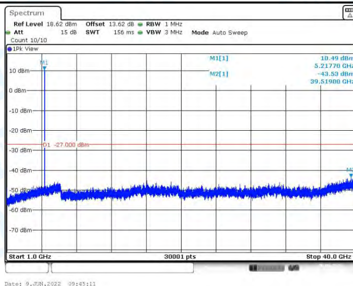
11AX20MIMO_Ant2_5220_1000~40000
