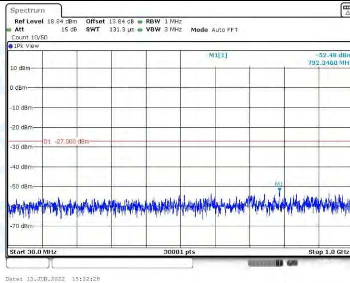
11AX20MIMO_Ant2_5260_30~1000
