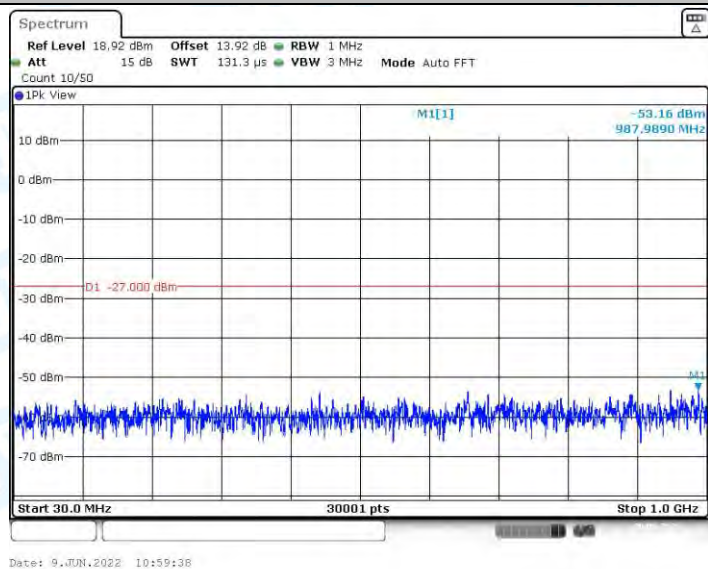
11AX40MIMO_Ant1_5795_30~1000
