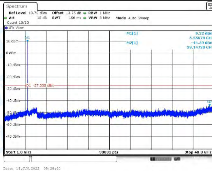
11AX20MIMO_Ant1_5260_1000~40000
