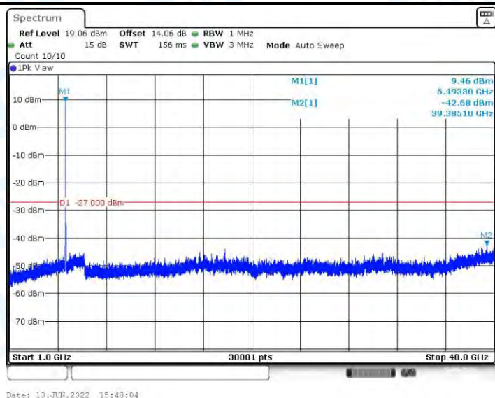
11AX20MIMO_Ant1_5500_1000~40000
