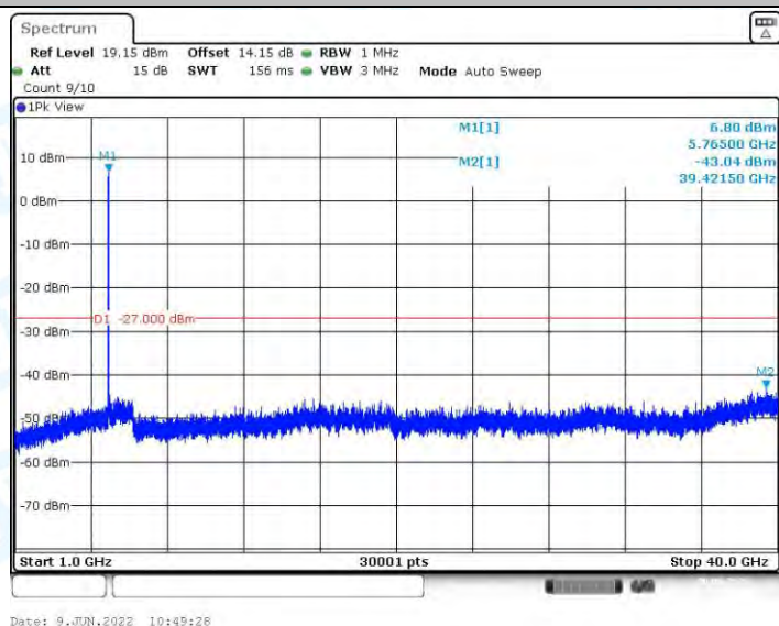
11AX40MIMO_Ant1_5755_1000~40000
