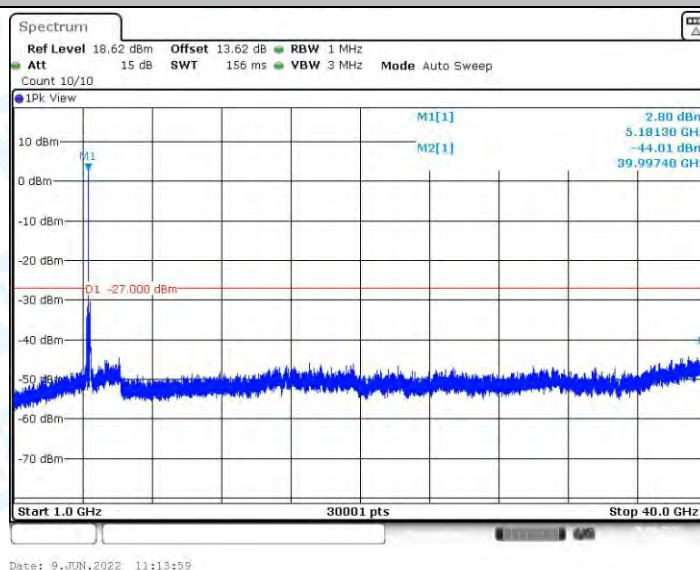
11AX80MIMO_Ant2_5210_1000~40000
