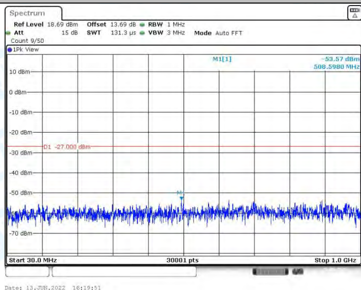
11AX40MIMO_Ant1_5270_30~1000
