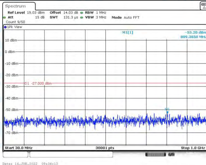
11AX40MIMO_Ant1_5510_30~1000
