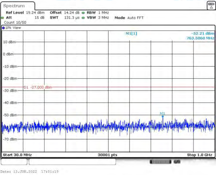
11AX80MIMO_Ant1_5530_30~1000
