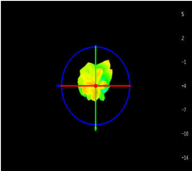
24250MHz
