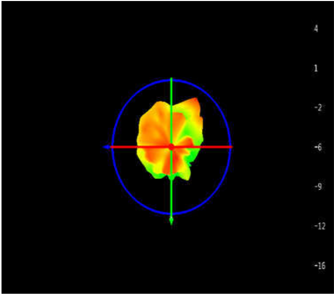
24150MHz
