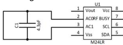
RFID Tag Schematic
