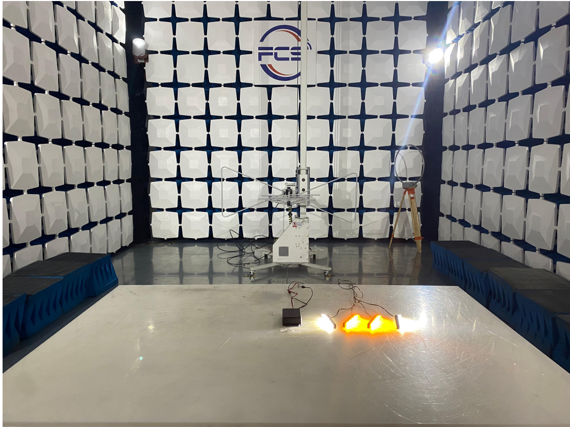
RE (Below1GHz)
