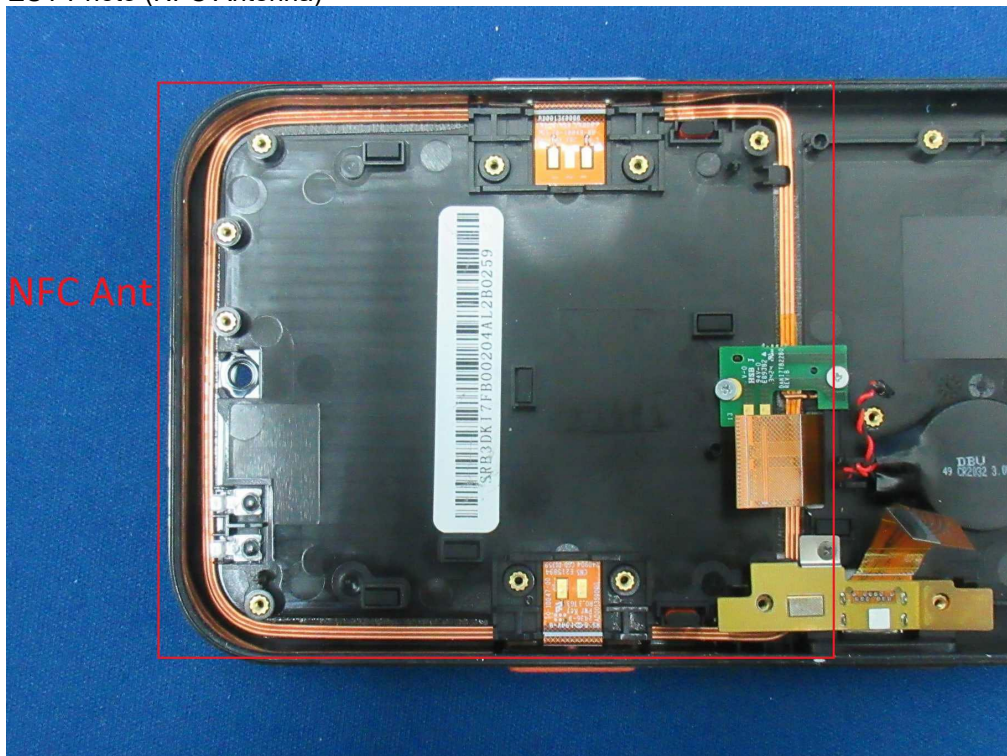
(22) EUT Photo (NFC Antenna)
