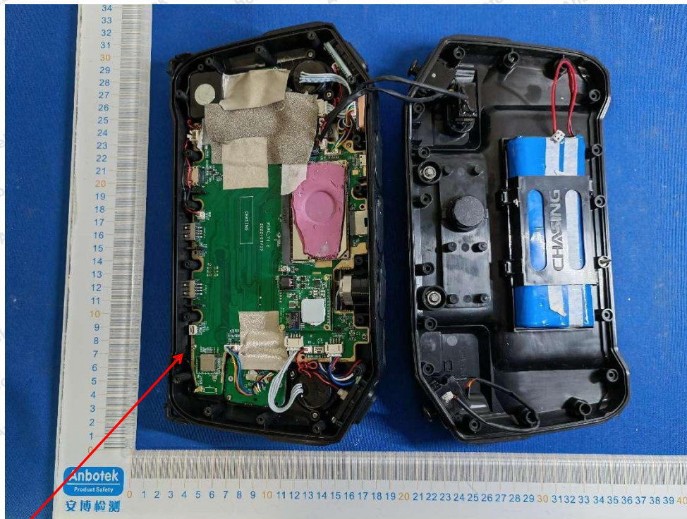
BT&WIFI ANT
