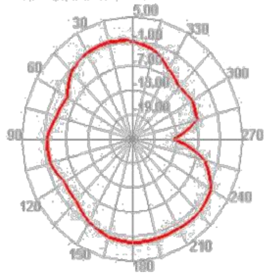
2400.000MHz E1
