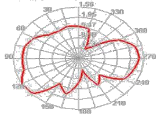
2400.000MHz E1
