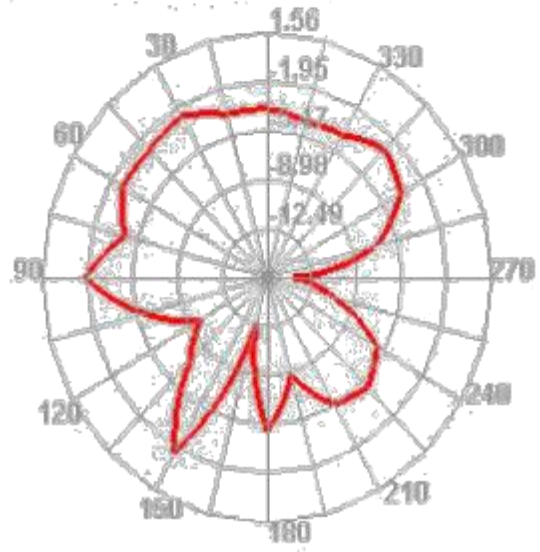
2400.000MHz E2
