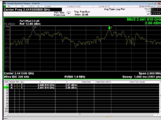
GFSK
