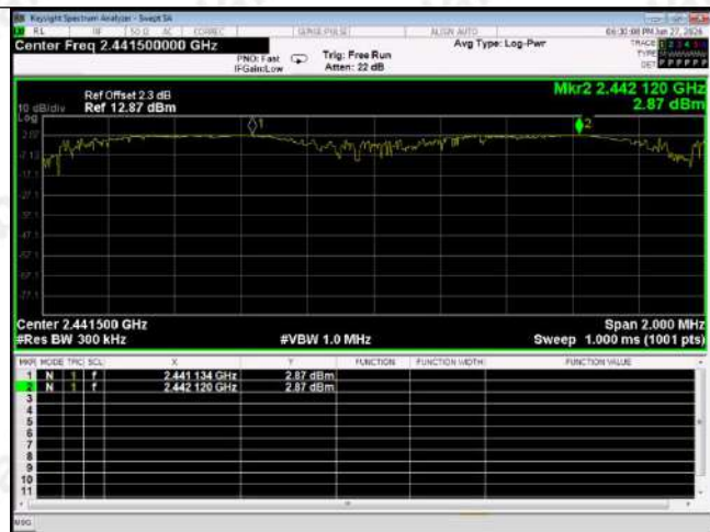
\pi/4 DQPSK
