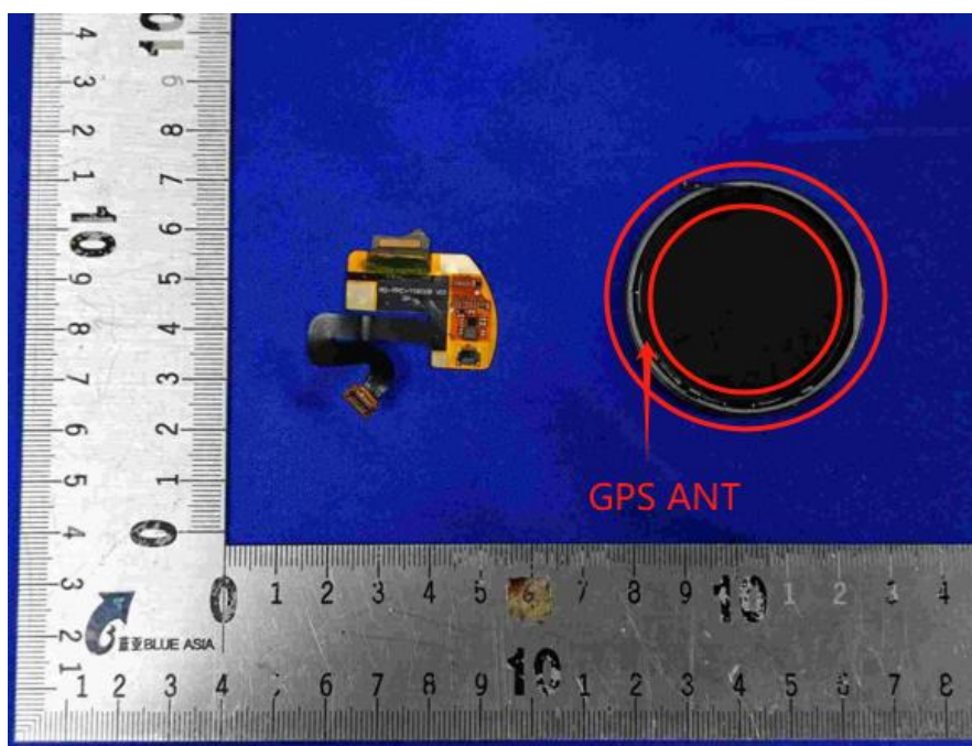
GPS ANT
