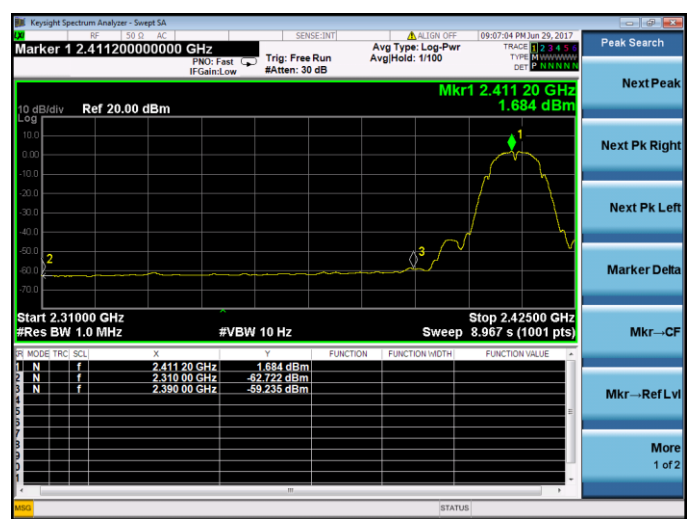
802.11b-Low channel(Average)
