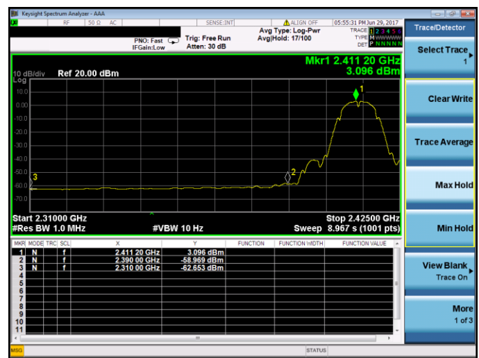
802.11b-Low channel(Average)
