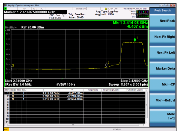
802.11g-Low channel(Average)
