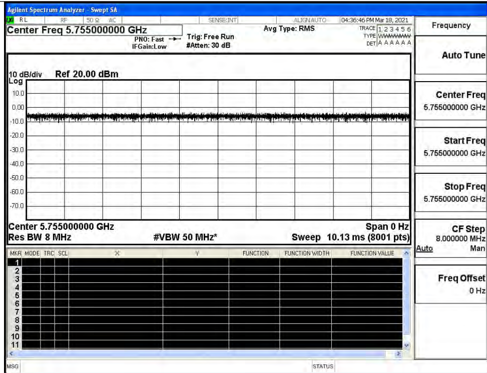
IEEE 802.11AC40
