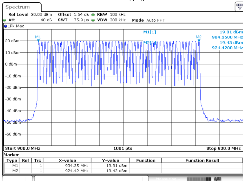
NVNT SRD Hopping Ant1
