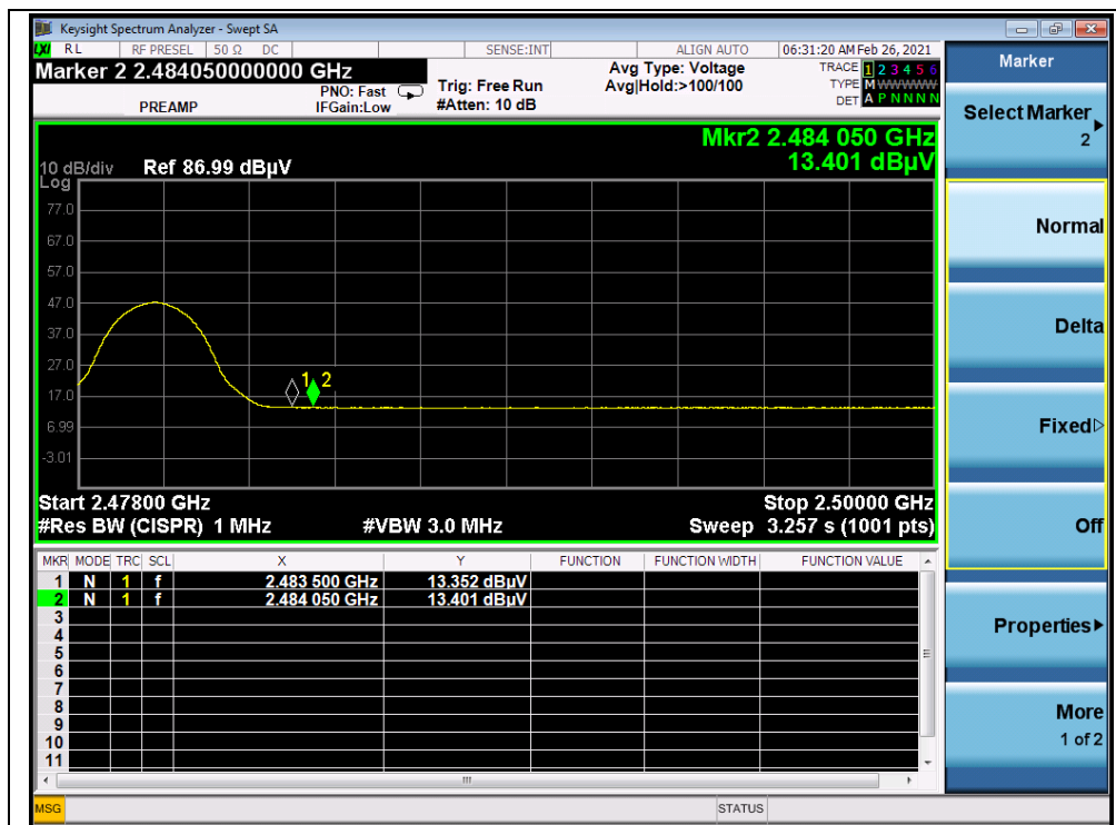
(AVERAGE, Channel 26)
