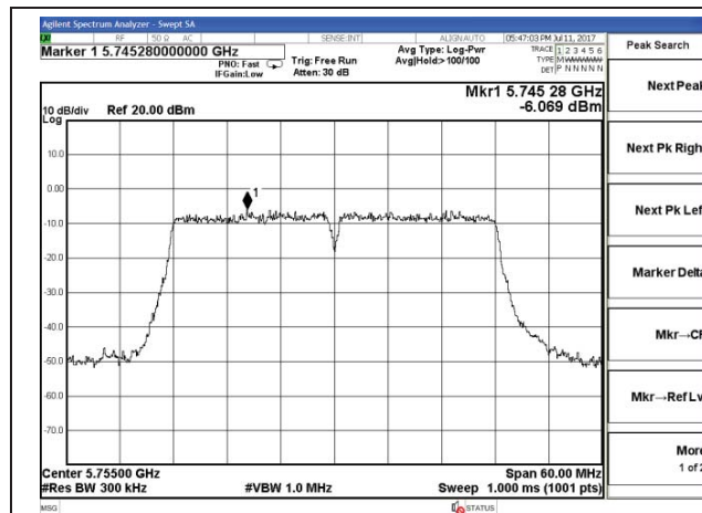
Chain 0-802.11n40-5755MHz
