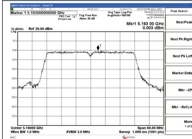
Chain 0-802.11n40-5190MHz
