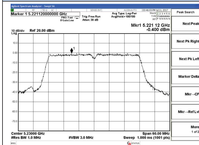
Chain 0-802.11n40-5230MHz
