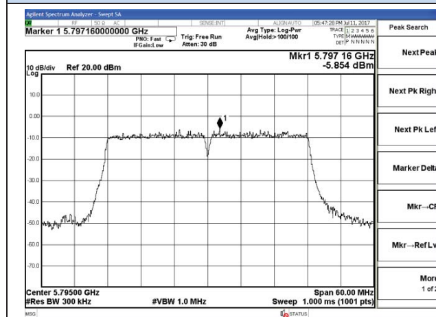
Chain 0-802.11n40-5795MHz
