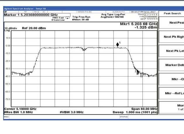
Chain 1-802.11n40-5190MHz
