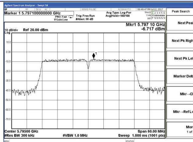
Chain 1-802.11n40-5795MHz
