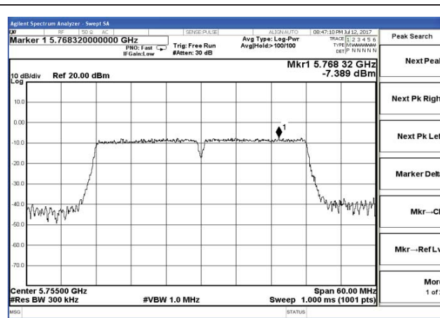
Chain 1-802.11n40-5755MHz
