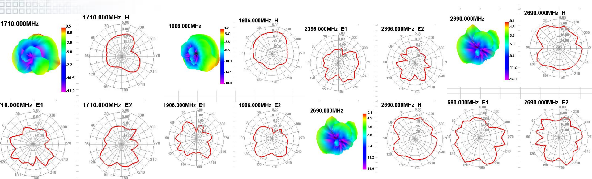
1710.00MHz - 2690.00MHz Gain
