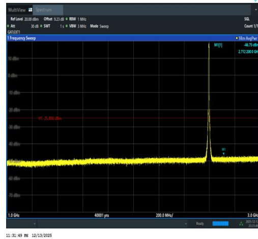
Band41(2535-2655)-5MHz-QPSK-40640-25RB# 0-1000~3000-PASS
