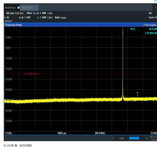
Band41(2535-2655)-5MHz-16QAM-40065-1RB#
