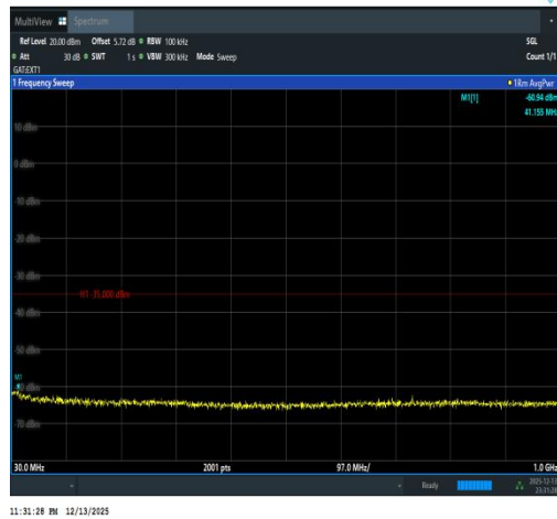
Band41(2535-2655)-5MHz-QPSK-40640-25RB# 0-30~1000-PASS
