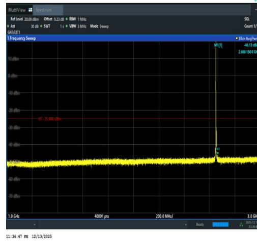
Band41(2535-2655)-5MHz-QPSK-41215-1RB#0-1000~3000-PASS
