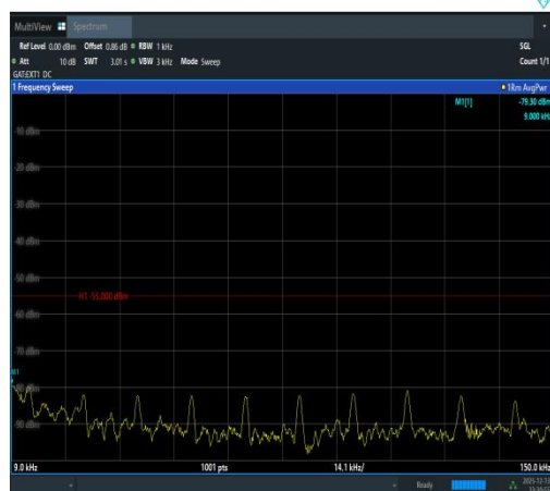
Band41(2535-2655)-5MHz-QPSK-40640-25RB#
