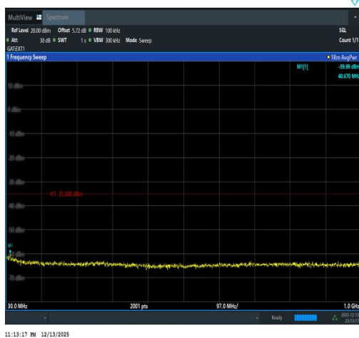
Band41(2535-2655)-5MHz-16QAM-40065-1RB#
