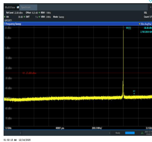
Band41(2535-2655)-10MHz-QPSK-40640-1RB# 49-1000~3000-PASS
