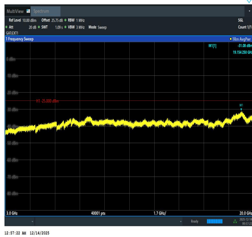
Band41(2535-2655)-10MHz-QPSK-40640-1RB# 0-3000~20000-PASS
