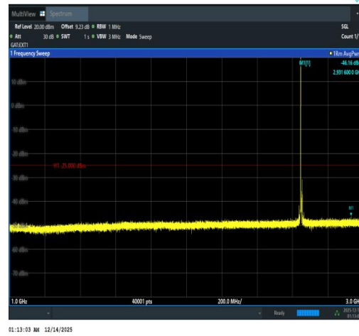
Band41(2535-2655)-10MHz-QPSK-41190-1RB# 0-1000~3000-PASS
