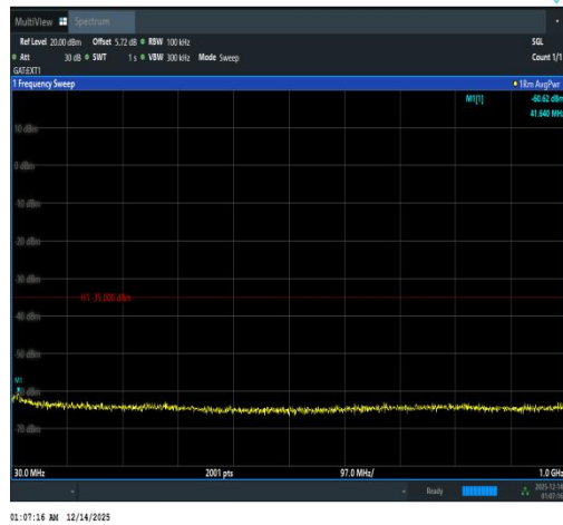
Band41(2535-2655)-10MHz-QPSK-40640-50RB #0-30~1000-PASS
