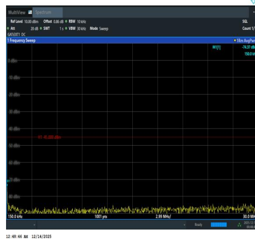
Band41(2535-2655)-10MHz-16QAM-40090-1RB
