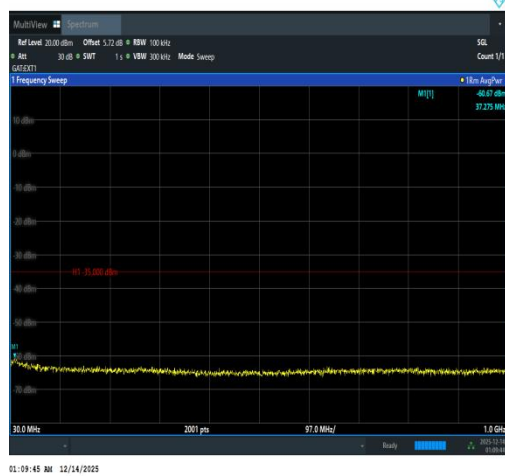
Band41(2535-2655)-10MHz-16QAM-40640-50R B#0-30~1000-PASS
