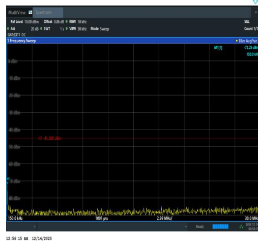
Band41(2535-2655)-10MHz-QPSK-40640-1RB#
