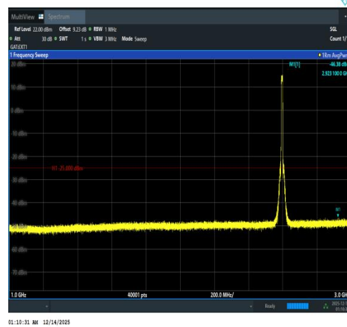
Band41(2535-2655)-10MHz-16QAM-40640-50R B#0-1000~3000-PASS
