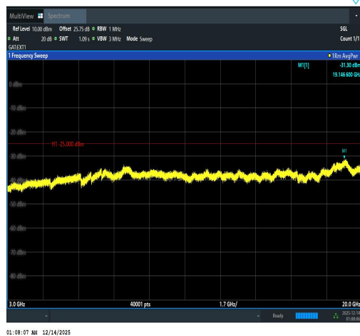
Band41(2535-2655)-10MHz-QPSK-40640-50RB #0-3000~20000-PASS
