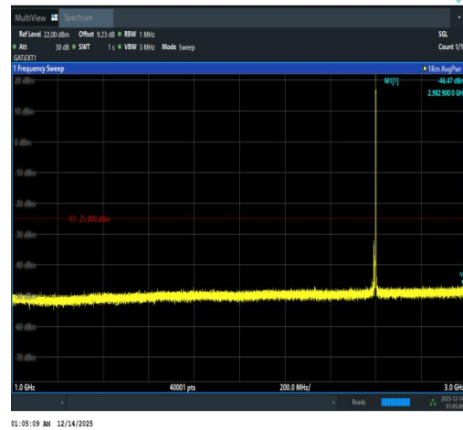
Band41(2535-2655)-10MHz-16QAM-40640-1RB #49-1000~3000-PASS
