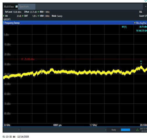
Band41(2535-2655)-10MHz-QPSK-41190-1RB# 0-3000~20000-PASS
