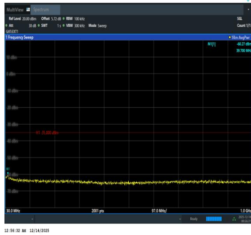
Band41(2535-2655)-10MHz-QPSK-40640-1RB# 0-30~1000-PASS
