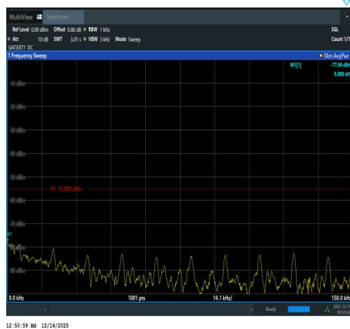
Band41(2535-2655)-10MHz-QPSK-40090-50RB
