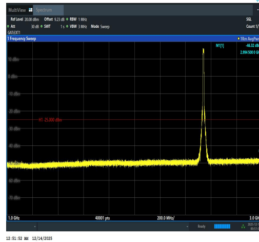
Band41(2535-2655)-10MHz-QPSK-40090-50RB #0-1000~3000-PASS
