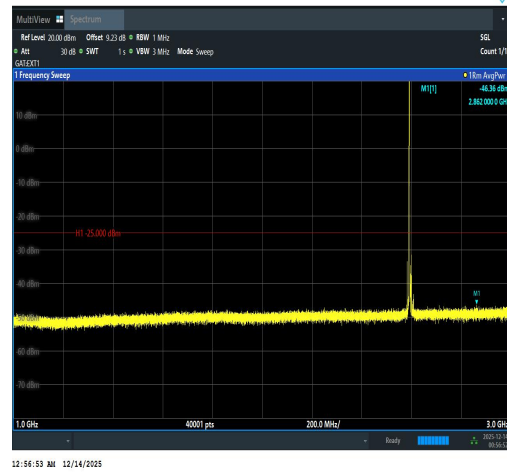
Band41(2535-2655)-10MHz-QPSK-40640-1RB# 0-1000~3000-PASS
