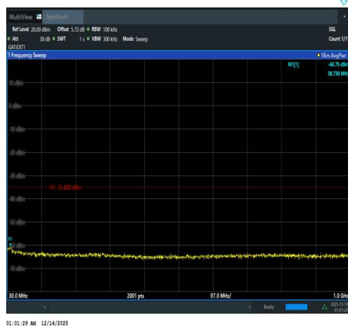
Band41(2535-2655)-10MHz-QPSK-40640-1RB# 49-30~1000-PASS
