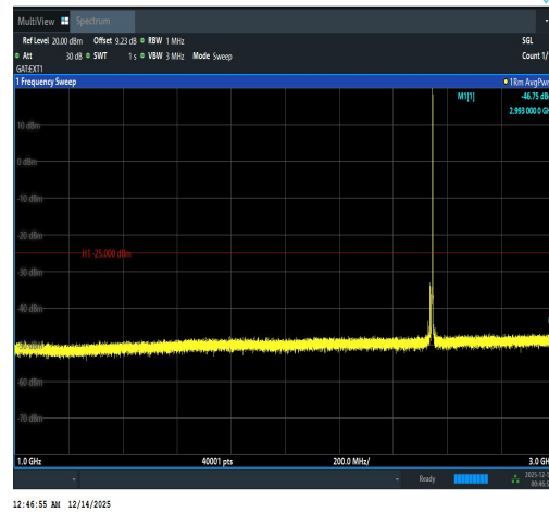
Band41(2535-2655)-10MHz-QPSK-40090-1RB# 49-1000~3000-PASS
