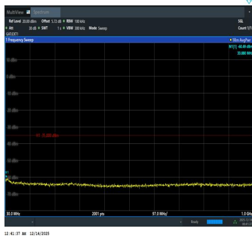
Band41(2535-2655)-10MHz-QPSK-40090-1RB# 0-30~1000-PASS
