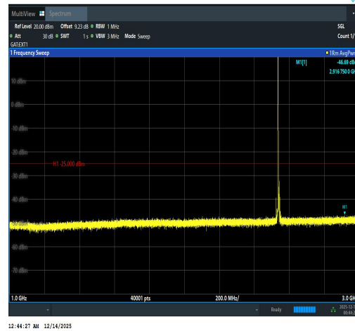
Band41(2535-2655)-10MHz-16QAM-40090-1RB #0-1000~3000-PASS
