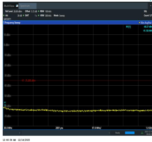
Band41(2535-2655)-10MHz-QPSK-40090-1RB# 49-30~1000-PASS
