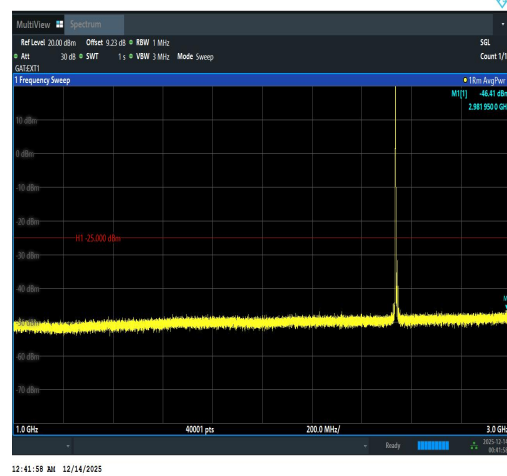
Band41(2535-2655)-10MHz-QPSK-40090-1RB# 0-1000~3000-PASS
