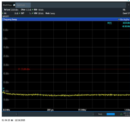
Band41(2535-2655)-10MHz-16QAM-40640-1RB #49-30~1000-PASS
