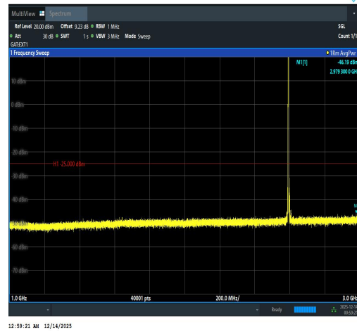
Band41(2535-2655)-10MHz-16QAM-40640-1RB #0-1000~3000-PASS
