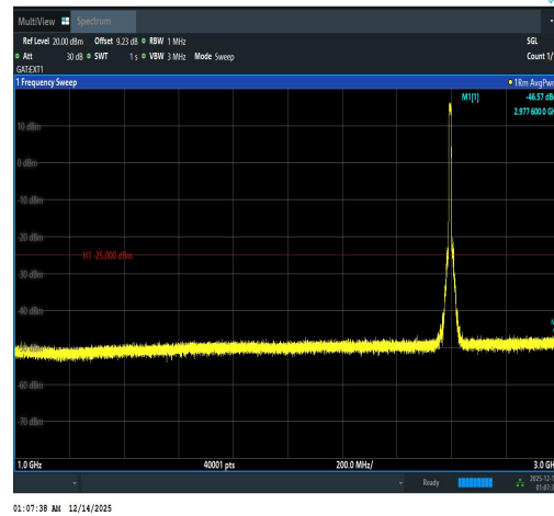
Band41(2535-2655)-10MHz-QPSK-40640-50RB #0-1000~3000-PASS
