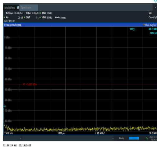
Band41(2535-2655)-15MHz-QPSK-41165-1RB#
