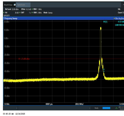
Band41(2535-2655)-20MHz-QPSK-40640-100R B#0-1000~3000-PASS
