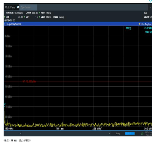
Band41(2535-2655)-15MHz-16QAM-41165-1RB
