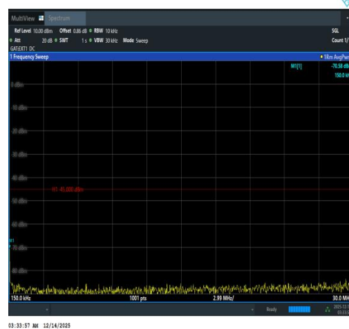
Band41(2535-2655)-20MHz-QPSK-40640-1RB#
