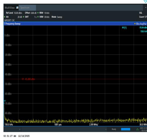
Band41(2535-2655)-15MHz-QPSK-41165-1RB#
