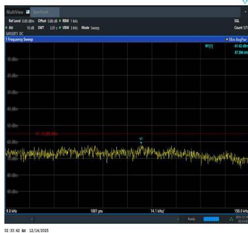
Band41(2535-2655)-15MHz-16QAM-41165-1RB
