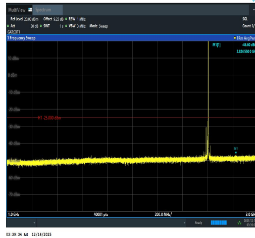
Band41(2535-2655)-20MHz-QPSK-40640-1RB# 99-1000~3000-PASS
