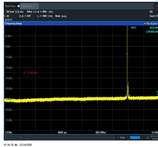
Band41(2535-2655)-20MHz-QPSK-40640-1RB# 0-1000~3000-PASS
