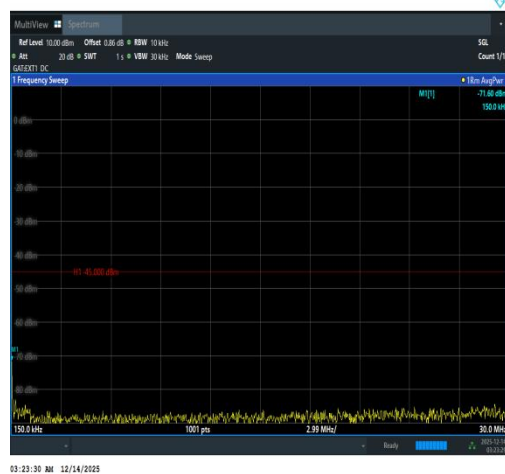
Band41(2535-2655)-20MHz-QPSK-40140-1RB#
