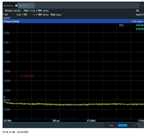
Band41(2535-2655)-20MHz-QPSK-40640-1RB# 0-30~1000-PASS
