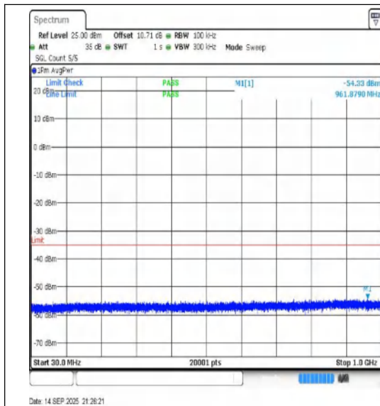
NTNV-n41-PC2-30-40-L-DFT-BPSK-Edge_1RB_L eft-30-1000-PASS
