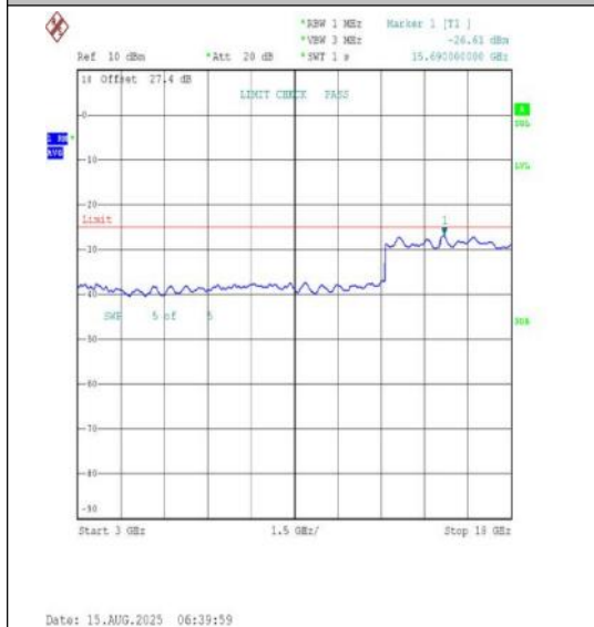
NTNV-n41-PC2-30-40-L-DFT-BPSK-Edge_1RB_L eft-3000-18000-PASS
