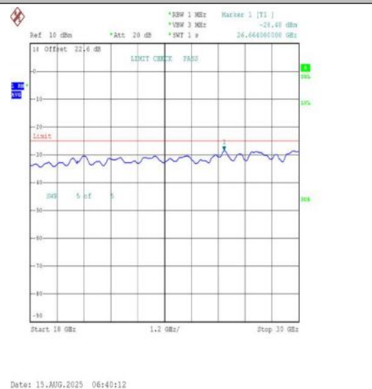
NTNV-n41-PC2-30-40-L-DFT-BPSK-Edge_1RB_L eft-18000-30000-PASS
