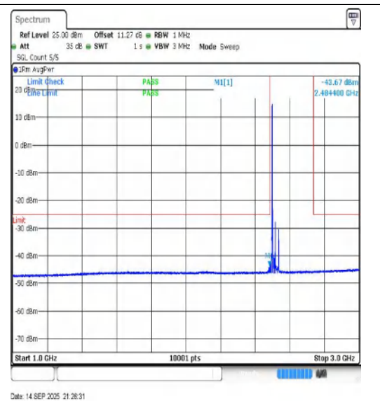
NTNV-n41-PC2-30-40-L-DFT-BPSK-Edge_1RB_L eft-1000-3000-PASS
