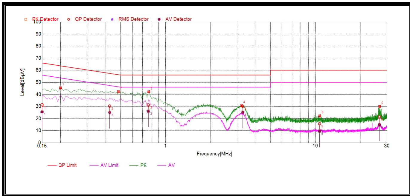
(Plot D: N Phase)
