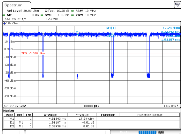
802.11n20_2437MHz
