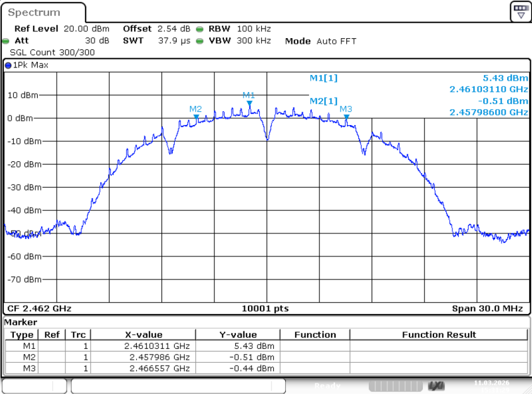
-6dB Bandwidth NVNT b 2462MHz Ant1
