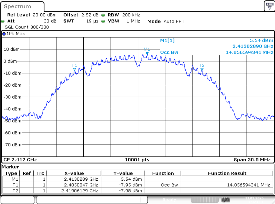
OBW NVNT b 2412MHz Ant1
