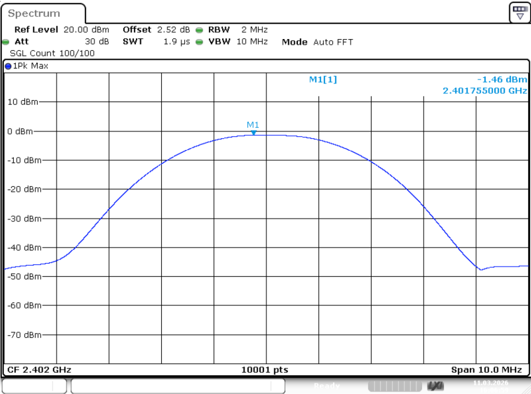
Peak Power NVNT BLE 1M 2402MHz Ant1
