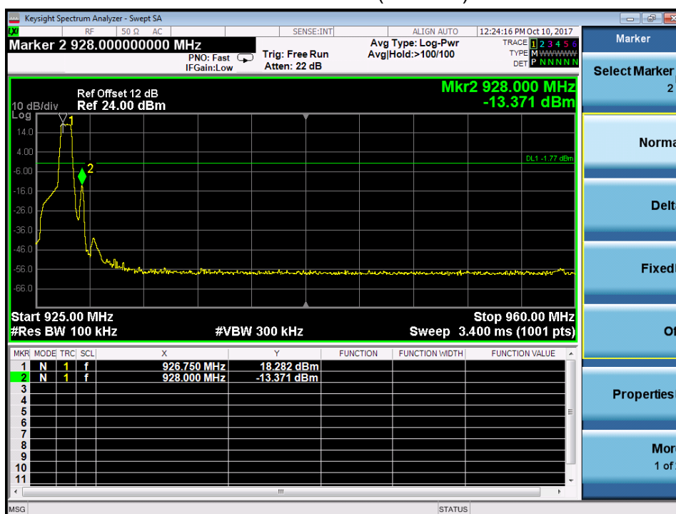
Mode 1 Channel(928MHz)
