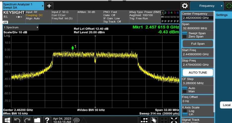
11G Ant1 2462
