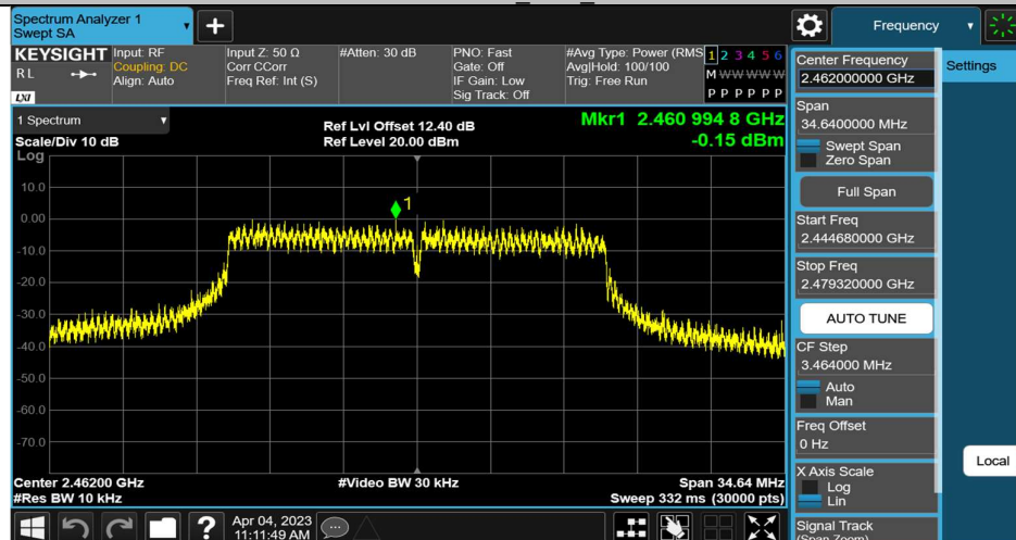
11N20SISO_Ant1_2462
