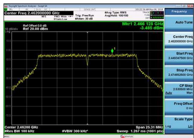
802.11g,2462MHz,Ant0
