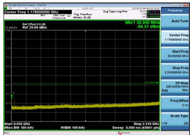
802.11n(HT40),2422MHz,Ant0,Plot 3,30MHz~2310MHz
