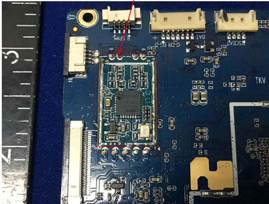
NFC Module
