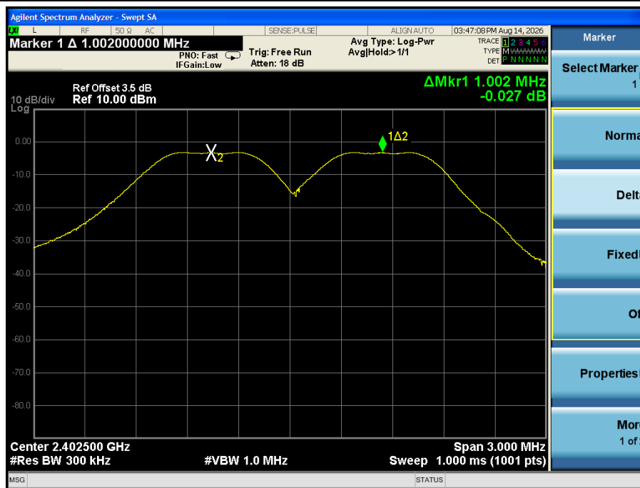
GFSK mode-CH00
