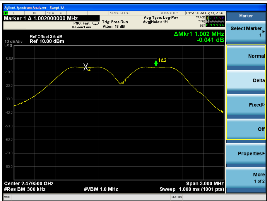
GFSK mode-CH78
