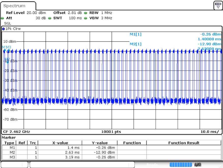
Test_Graph_802.11n20_ANT1_2462
