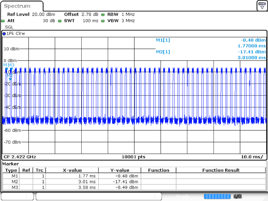
Test_Graph_802.11n40_ANT1_2422
