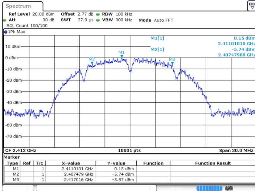
Test_Graph_802.11b_ANT1_2412
