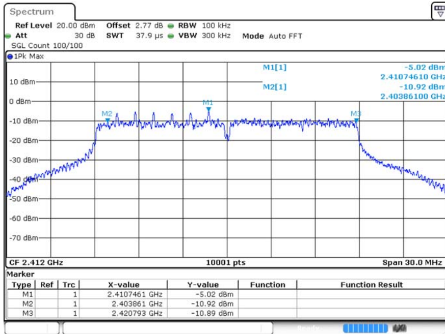
Test_Graph_802.11n20_ANT1_2412
