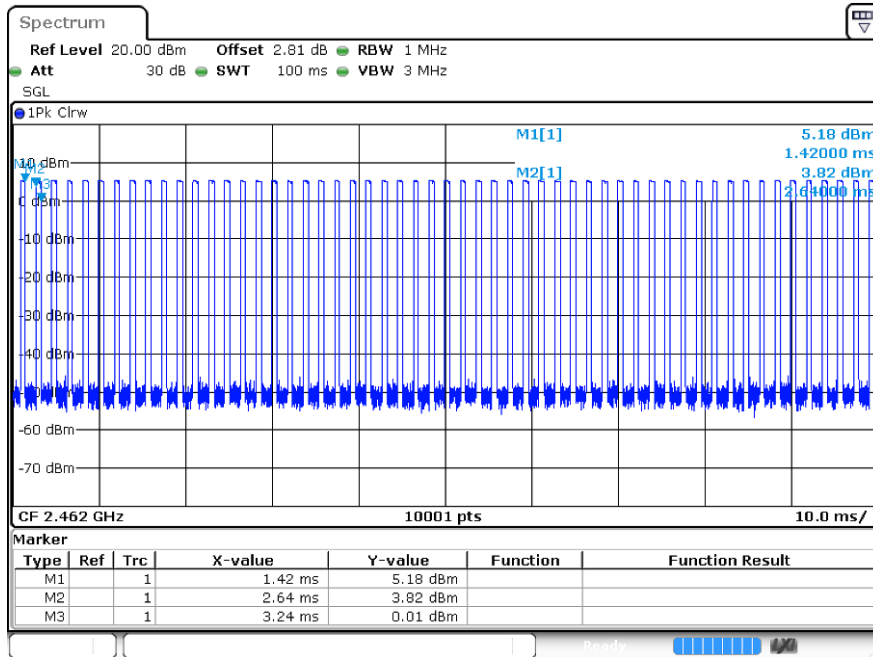
Test_Graph_802.11b_ANT1_2462
