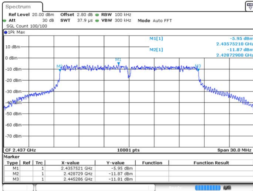
Test_Graph_802.11g_ANT1_2437
