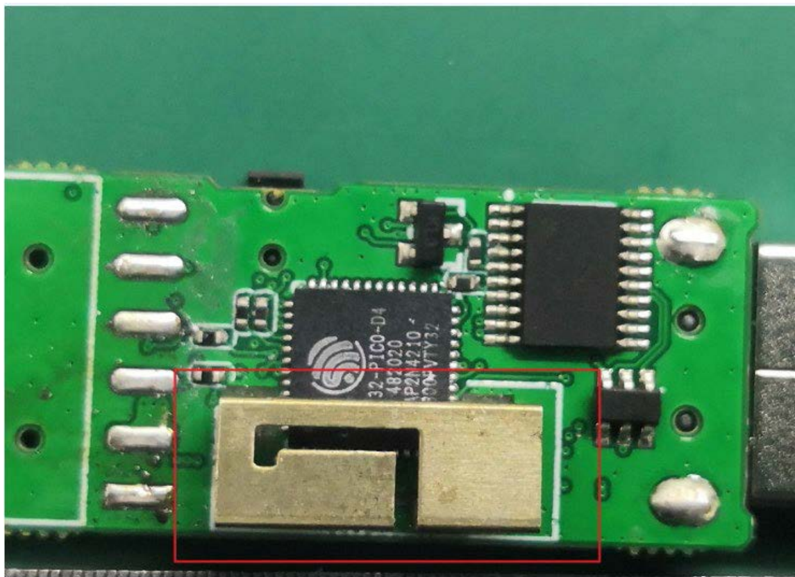
Antenna
