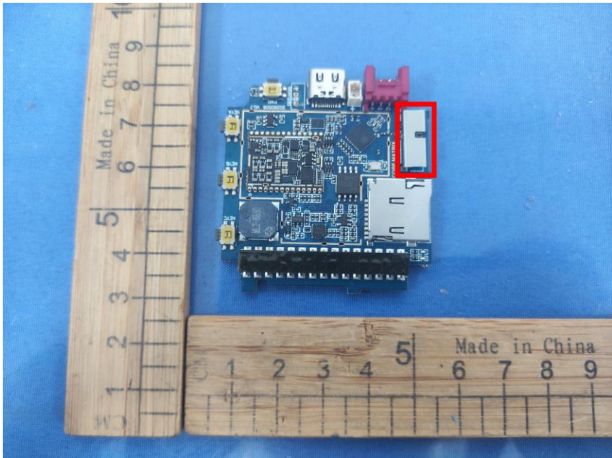
ANT
