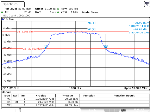
802.11ac20_5320MHz
