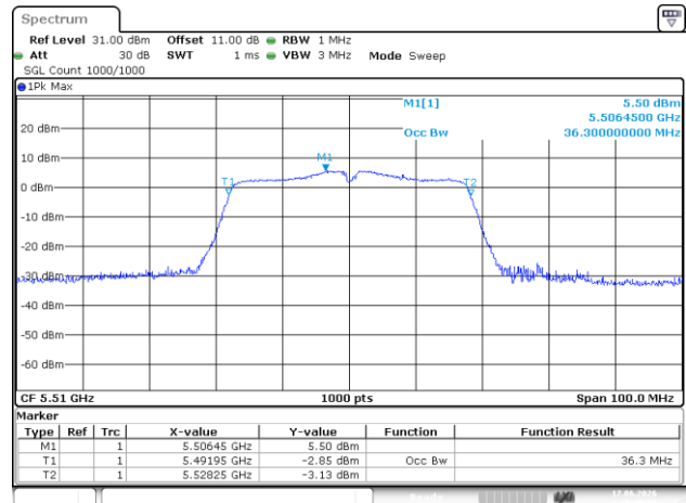
802.11n40_5510MHz
