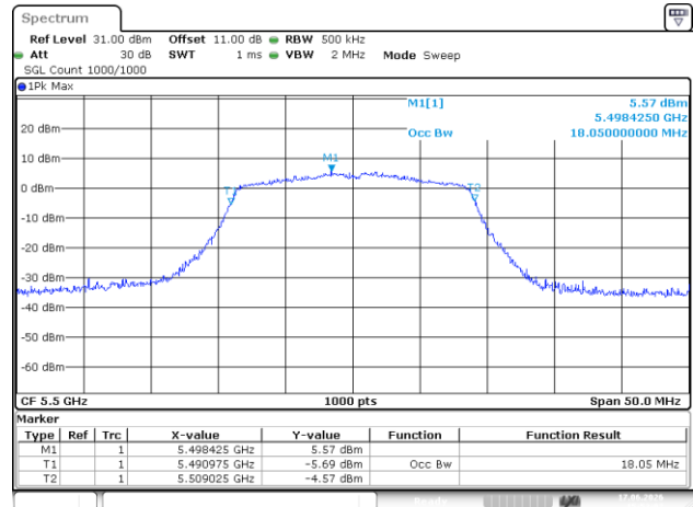
802.11ac20_5500MHz
