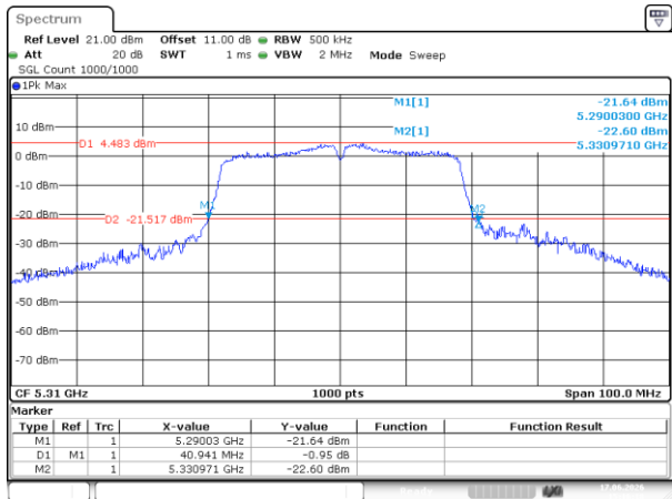
802.11n40_5310MHz
