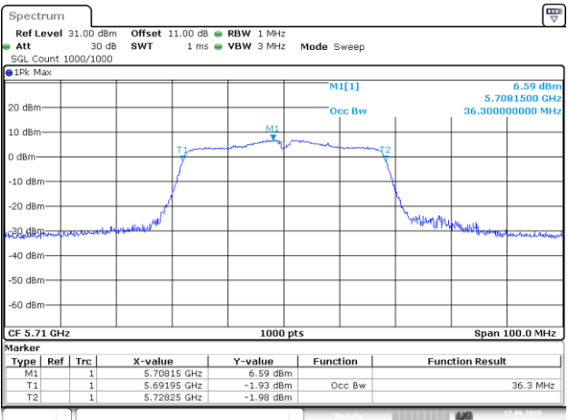
802.11n40_5710MHz
