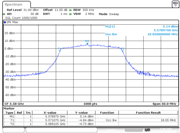
802.11n20_5580MHz
