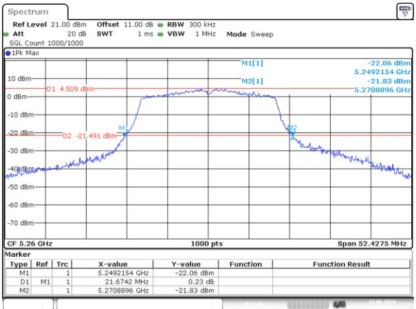
802.11ac20_5260MHz
