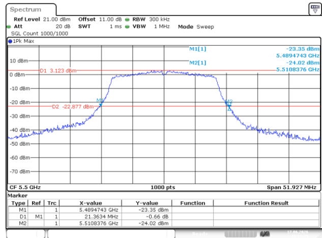
802.11ac20_5500MHz
