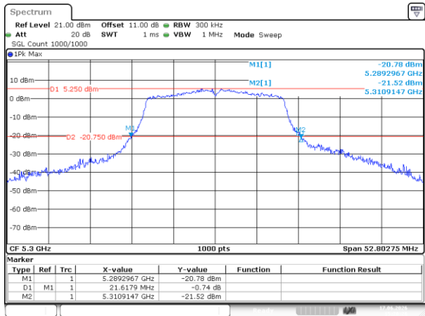
802.11ac20_5300MHz
