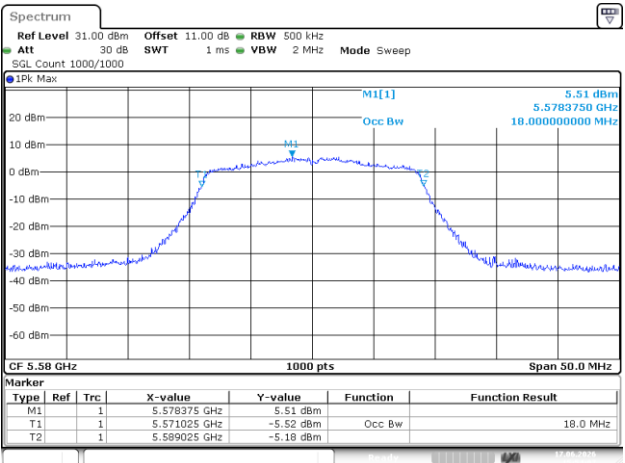
802.11ac20_5580MHz
