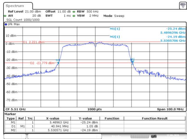
802.11n40_5510MHz
