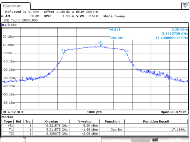
802.11a_5320MHz
