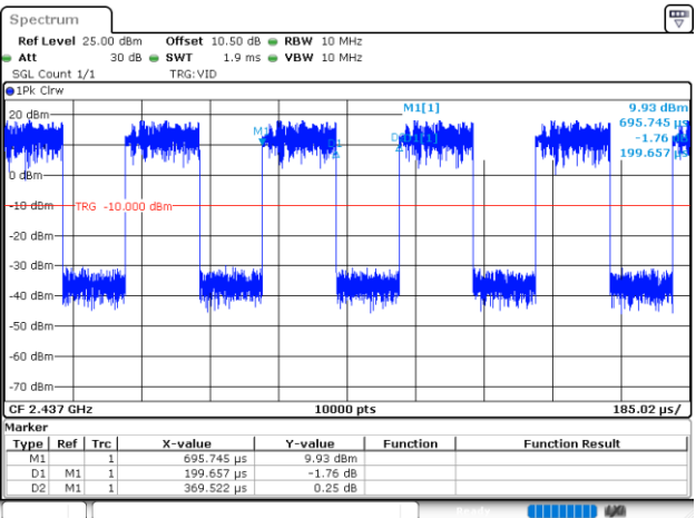
802.11n20_2437MHz
