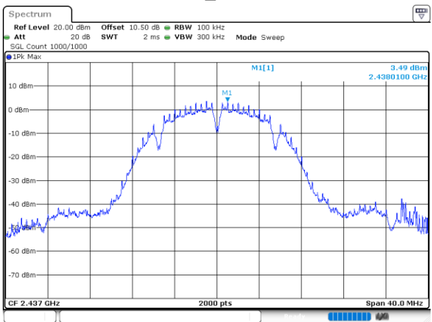
802.11b_2437MHz
