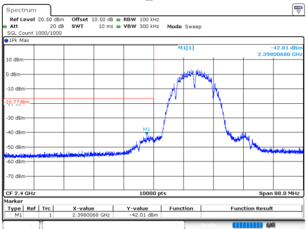
802.11b_2412MHz
