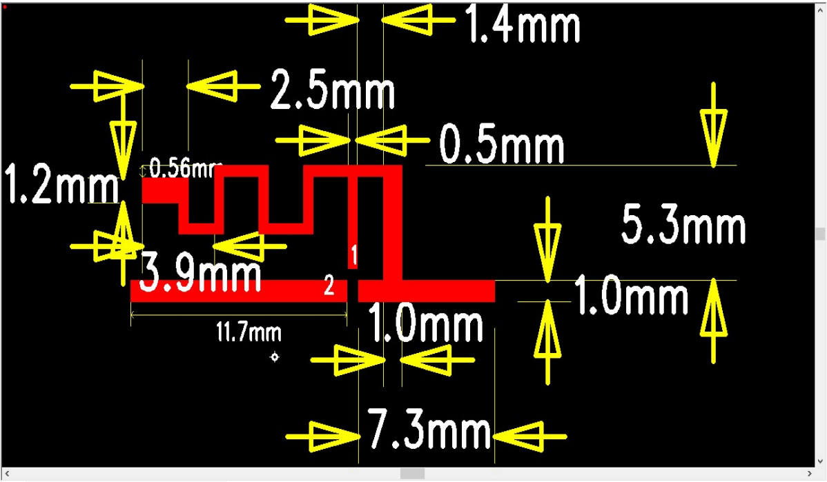
1、天线尺寸图
