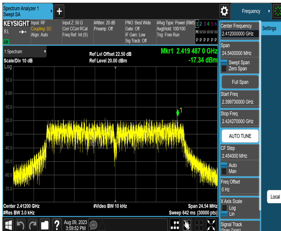
11G_Ant1_2412
