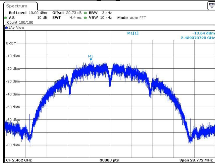
11B_Ant2_2462
