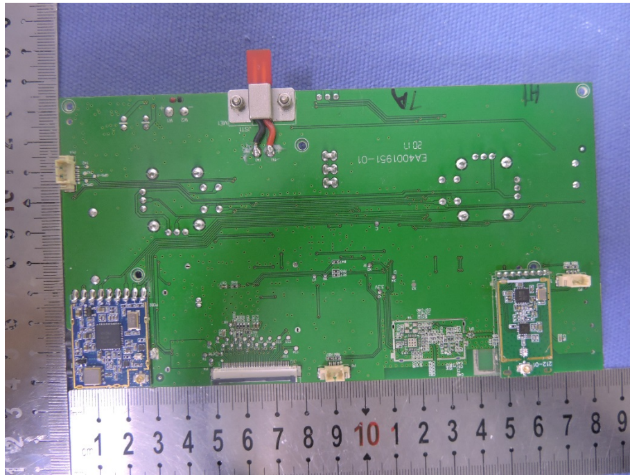
5.8GHz_ RX module
