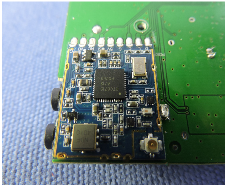
5.8GHz_ RX module
