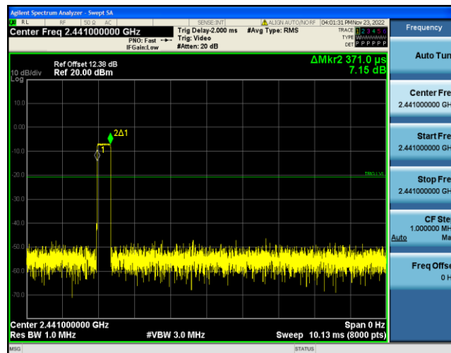
DH3-Ant1-Hop-1.620-160
