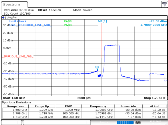
20MHz_Low_16QAM_25@0
