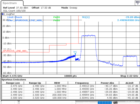
20MHz_Low_16QAM_25@0
