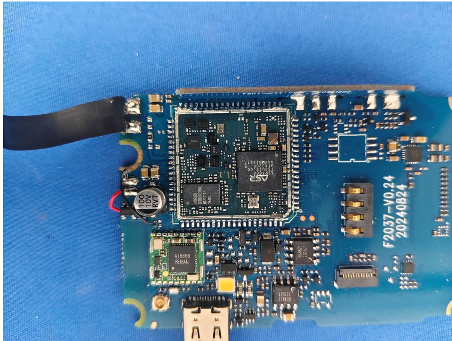
LTE Antenna
