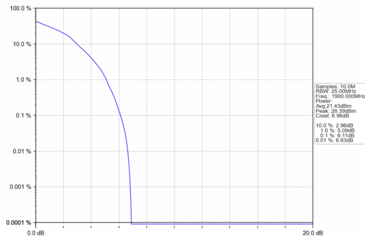
Band2 20MHz 16QAM HCH 1900MHz RB 27 73 NTNV
