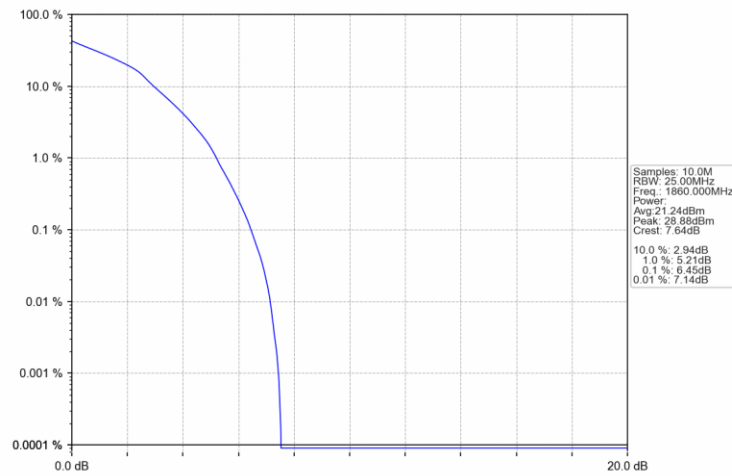
Band2_20MHz_16QAM_LCH_1860MHz_RB_27_0_NTNV
