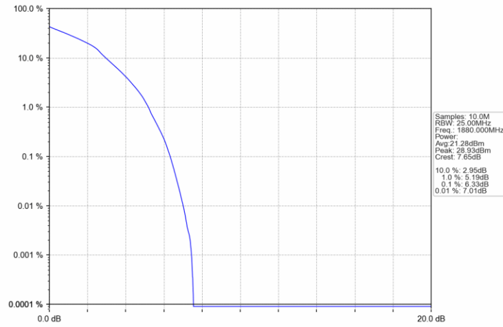
Band2 20MHz 16QAM MCH 1880MHz RB 27 0 NTNV
