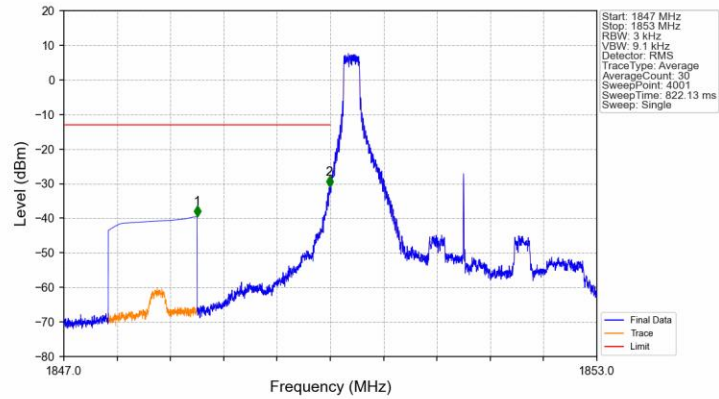
Band2_3MHz_QPSK_LCH_1851.5MHz_RB_1_0_NTNV
