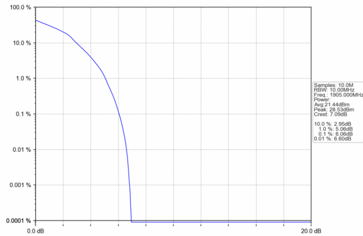
Band2_10MHz_16QAM_HCH_1905MHz_RB_27_23_NTNV
