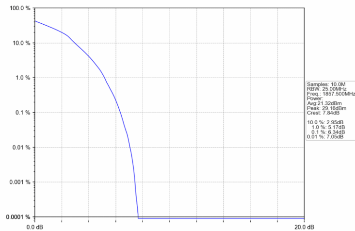
Band2 15MHz 16QAM LCH 1857.5MHz RB 27 0 NTNV
