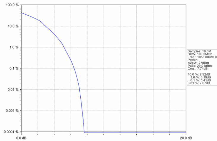
Band2 10MHz 16QAM LCH 1855MHz RB 27 0 NTV
